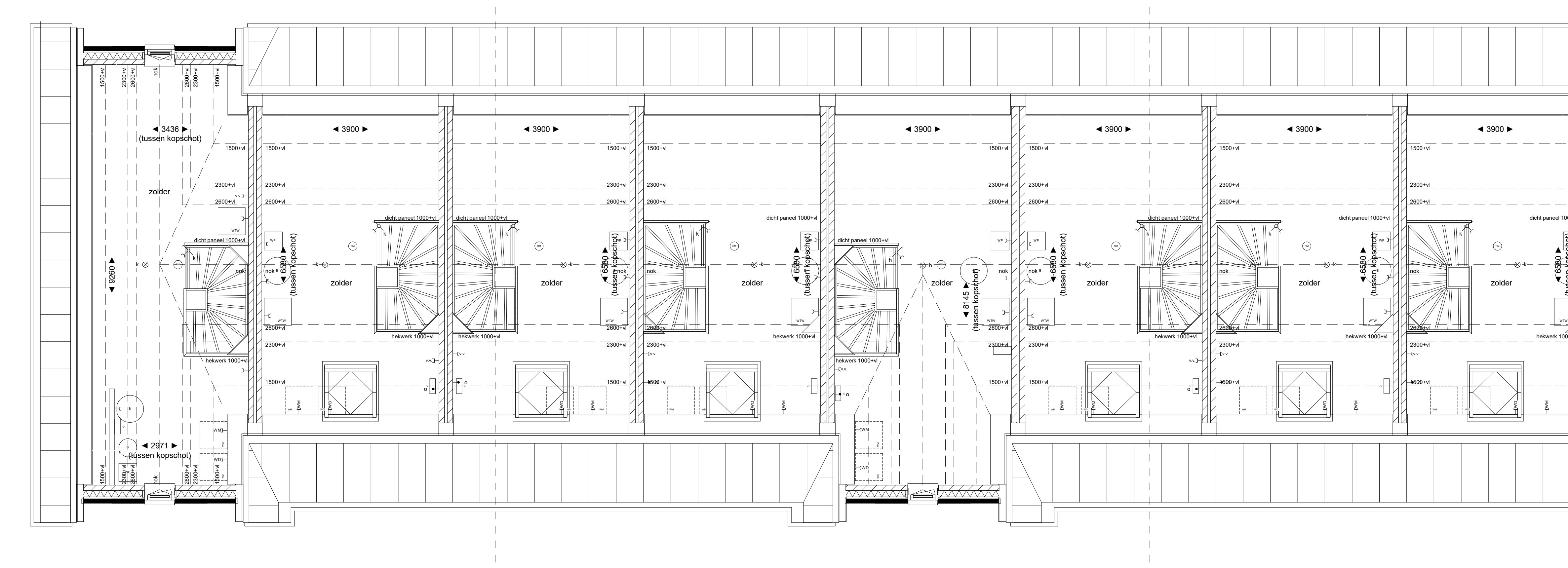
zolder 1:100 bwnr. 43 type G bwnr. 44a type H bwnr. 44b type H bwnr. 44c type H bwnr. 45 type I bwnr. 46a type H bwnr. 46b type H bwnr. 46c type H
