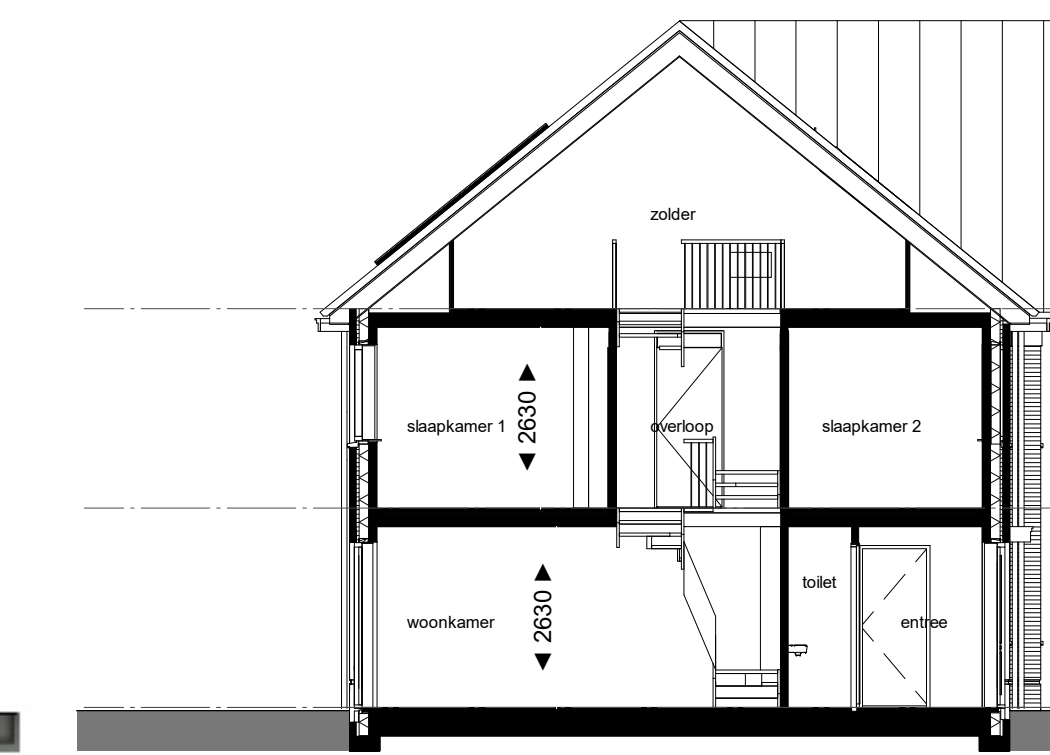
Doorsnede AA 1:100 bwnr. 44b type H
