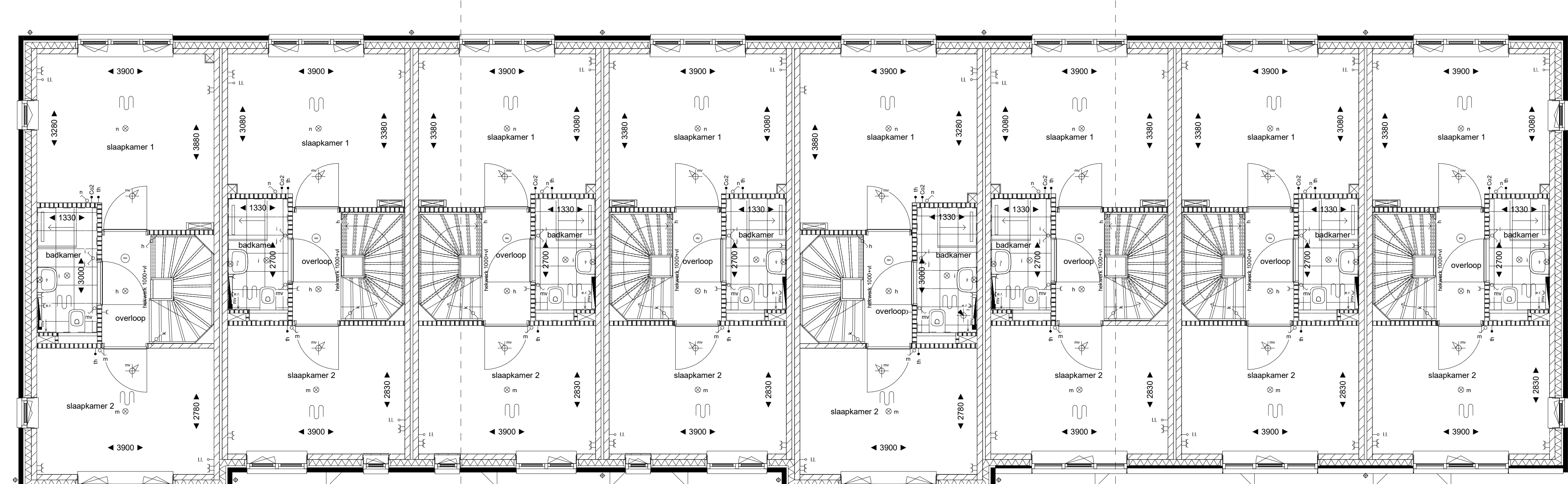
eerste verdieping 1:100 bwnr. 43 type G bwnr. 44a type H bwnr. 44b type H bwnr. 44c type H bwnr. 45 type I bwnr. 46a type H bwnr. 46b type H bwnr. 46c type H
