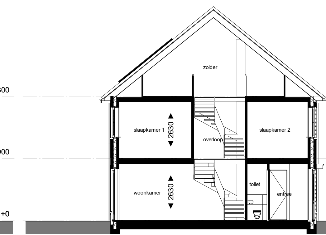
Doorsnede BB 1:100 bwnr. 46a type H
