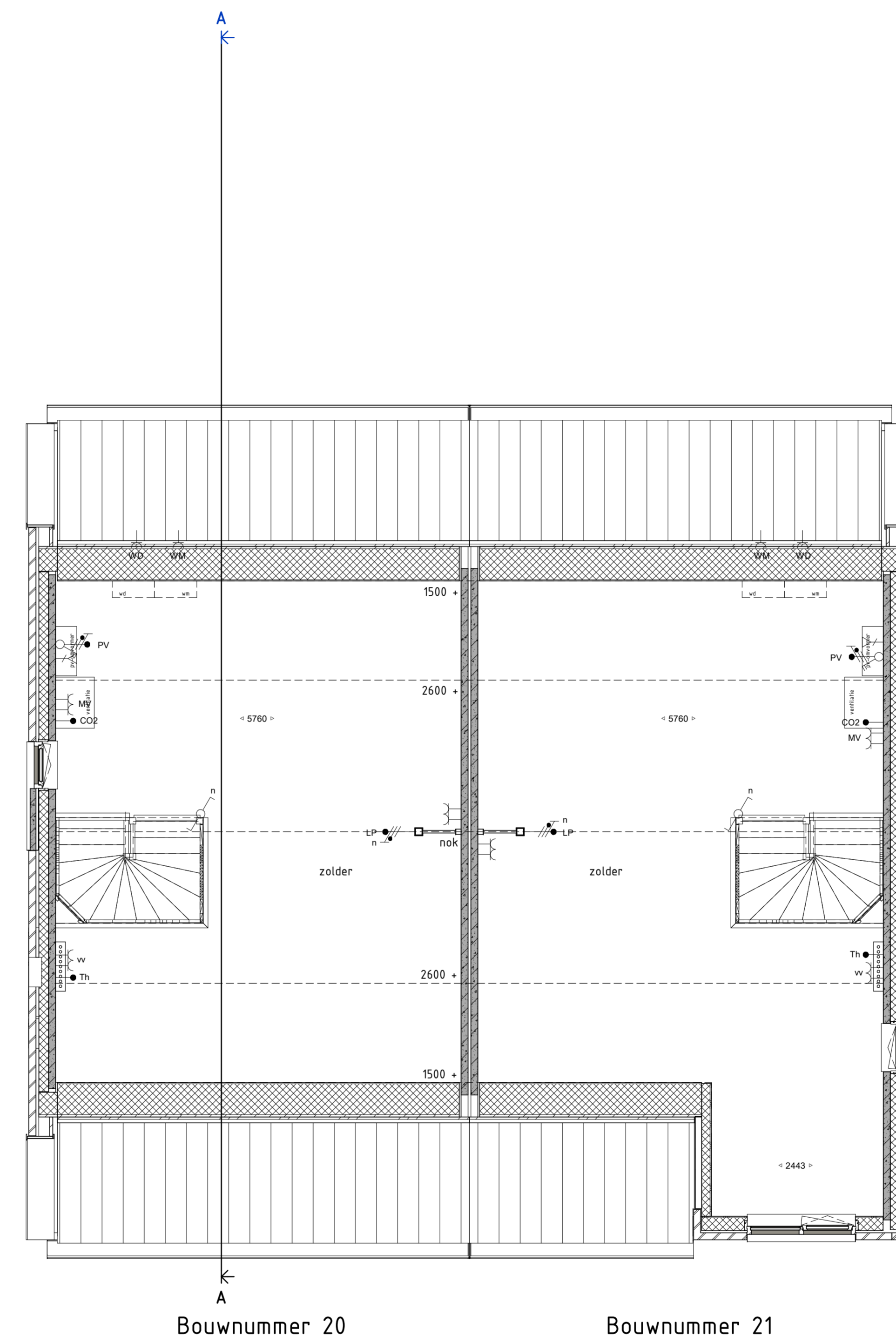
TWEDE VERDIEPING 1 : 50
