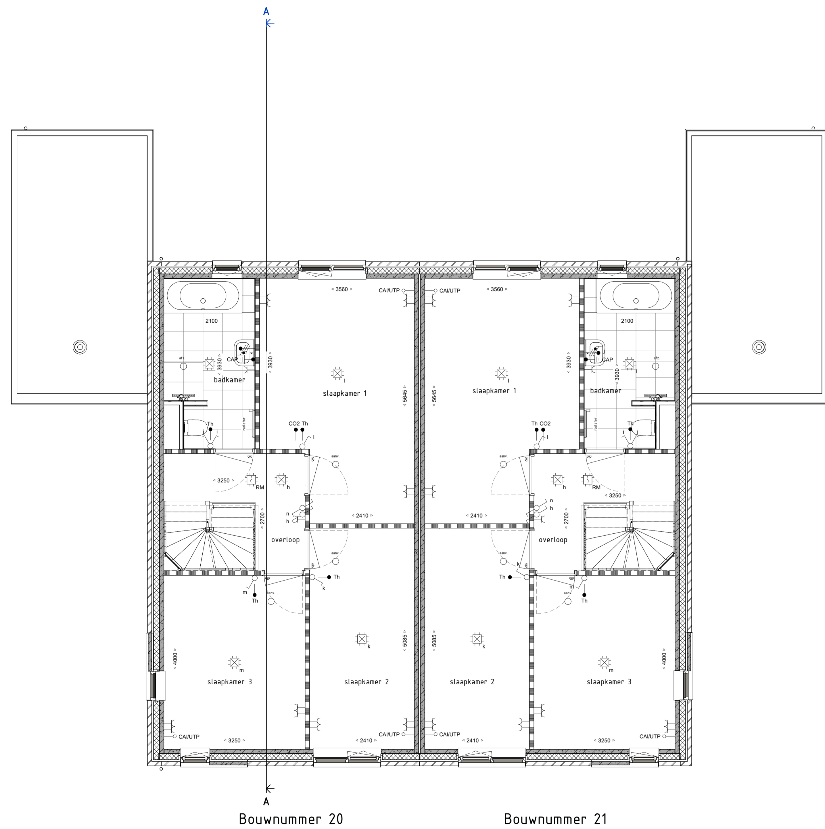
EERSTE VERDIEPING 1 : 50
