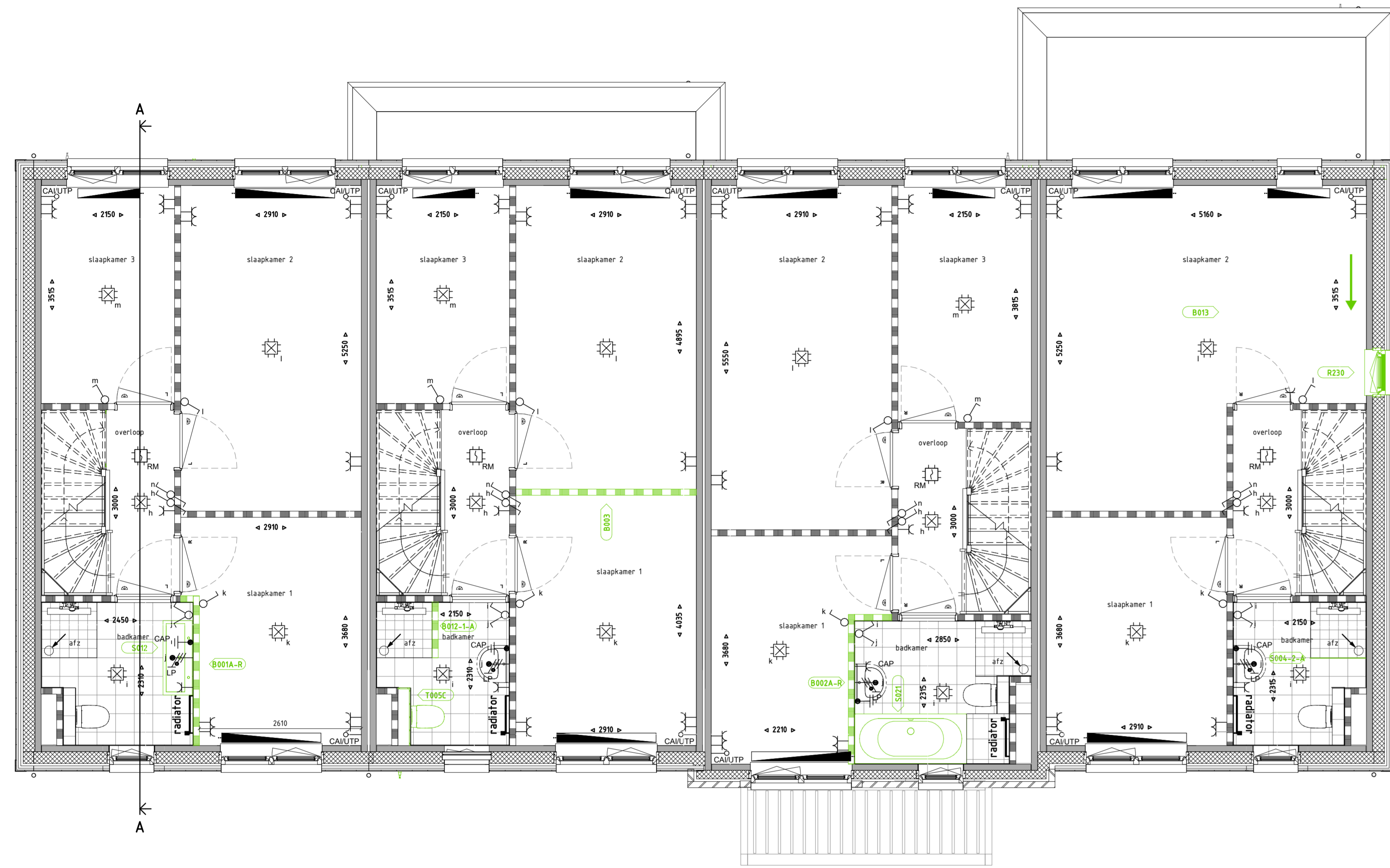
1E VERDIEPING 1 : 50
