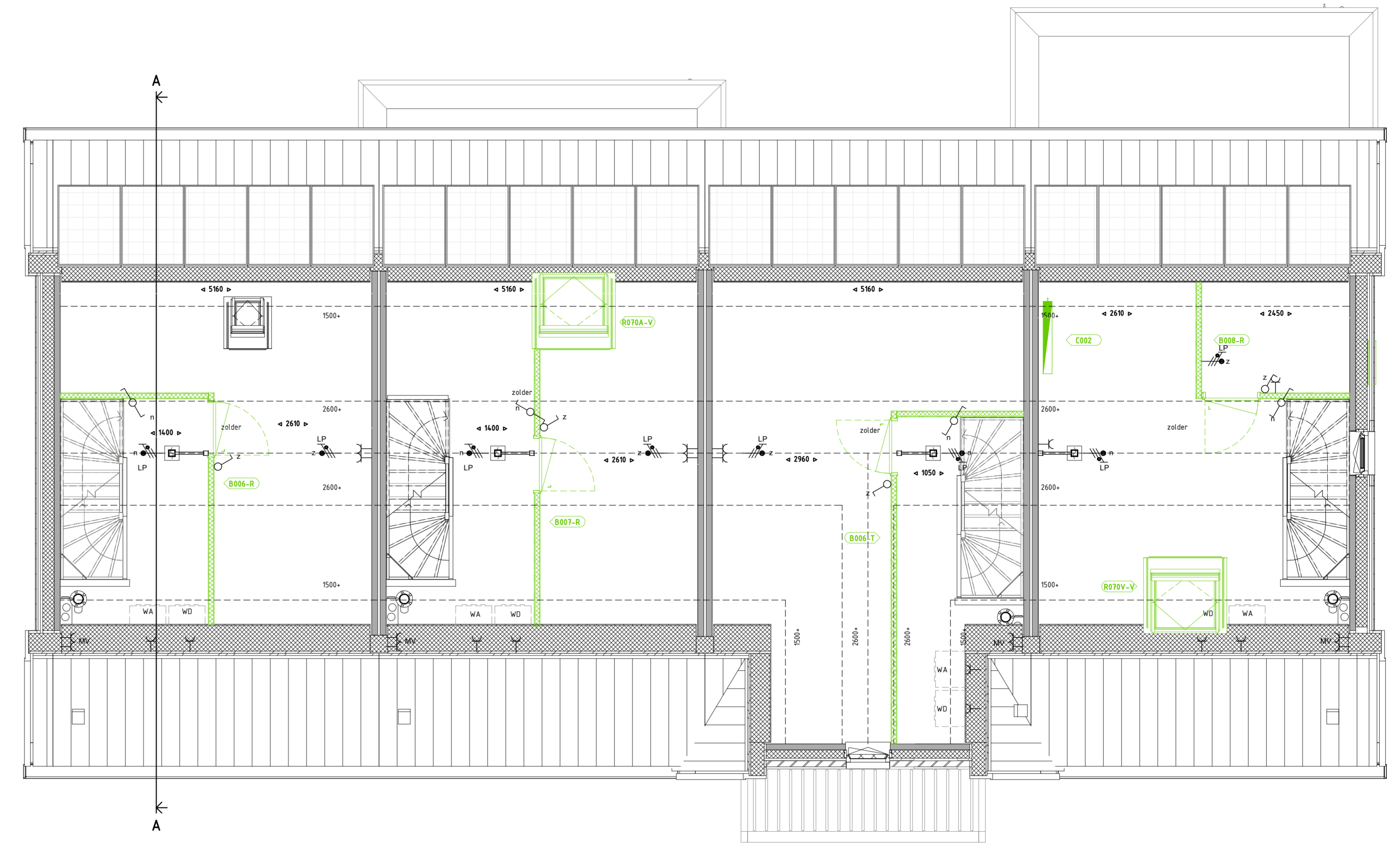
2E VERDIEPING 1 : 50
