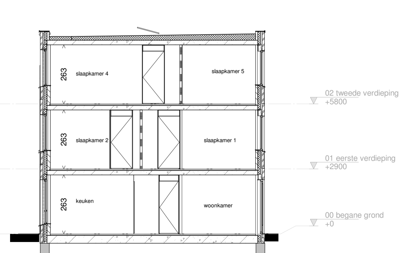
langdoorsnede 1 : 100
