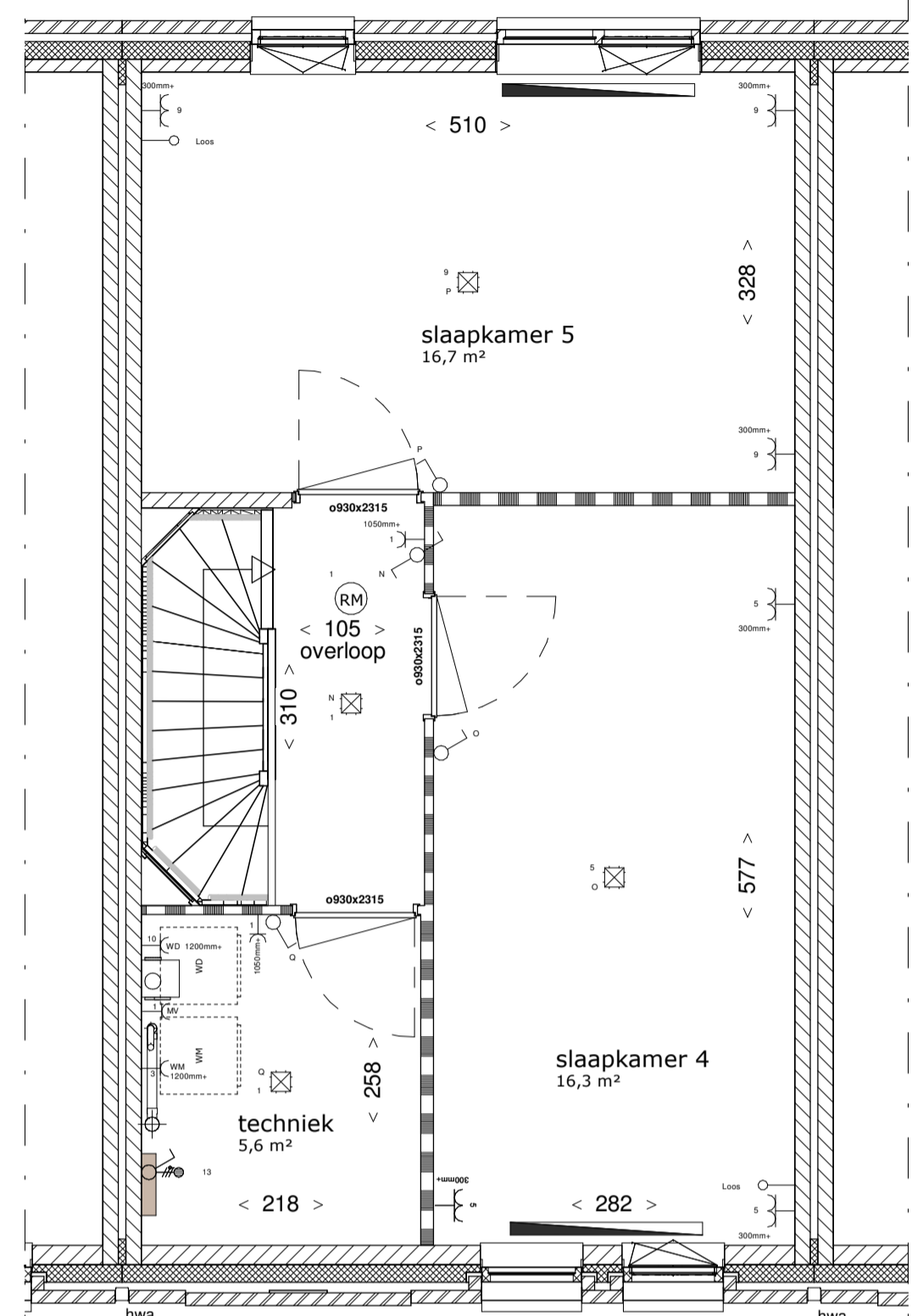
tweede verdieping 1 : 50
