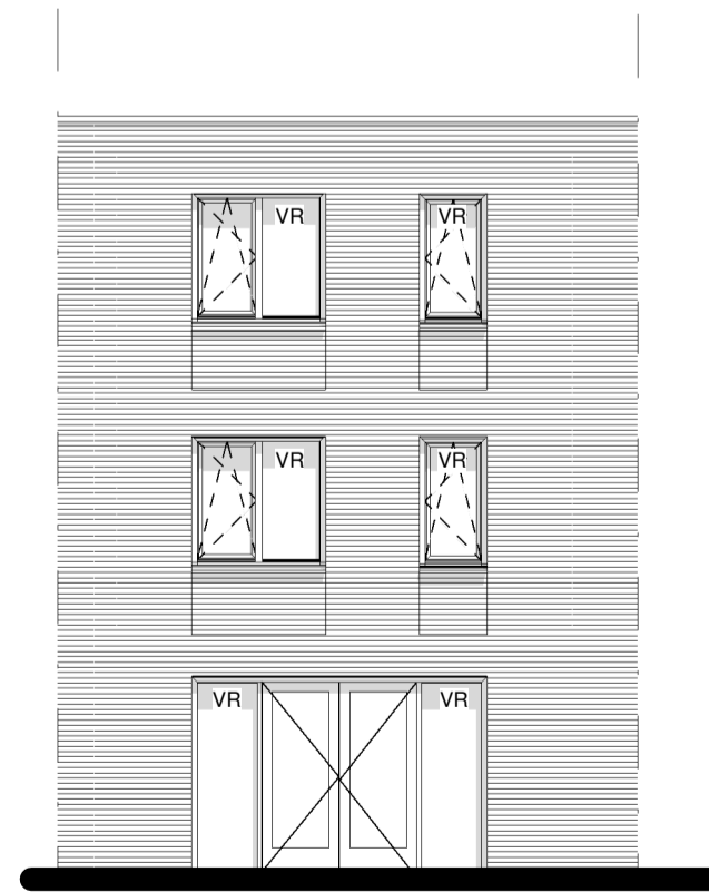
Achtergevel 1 : 100
