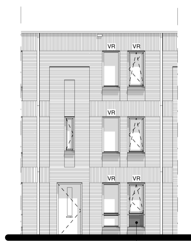
Voorgevel 1 : 100
