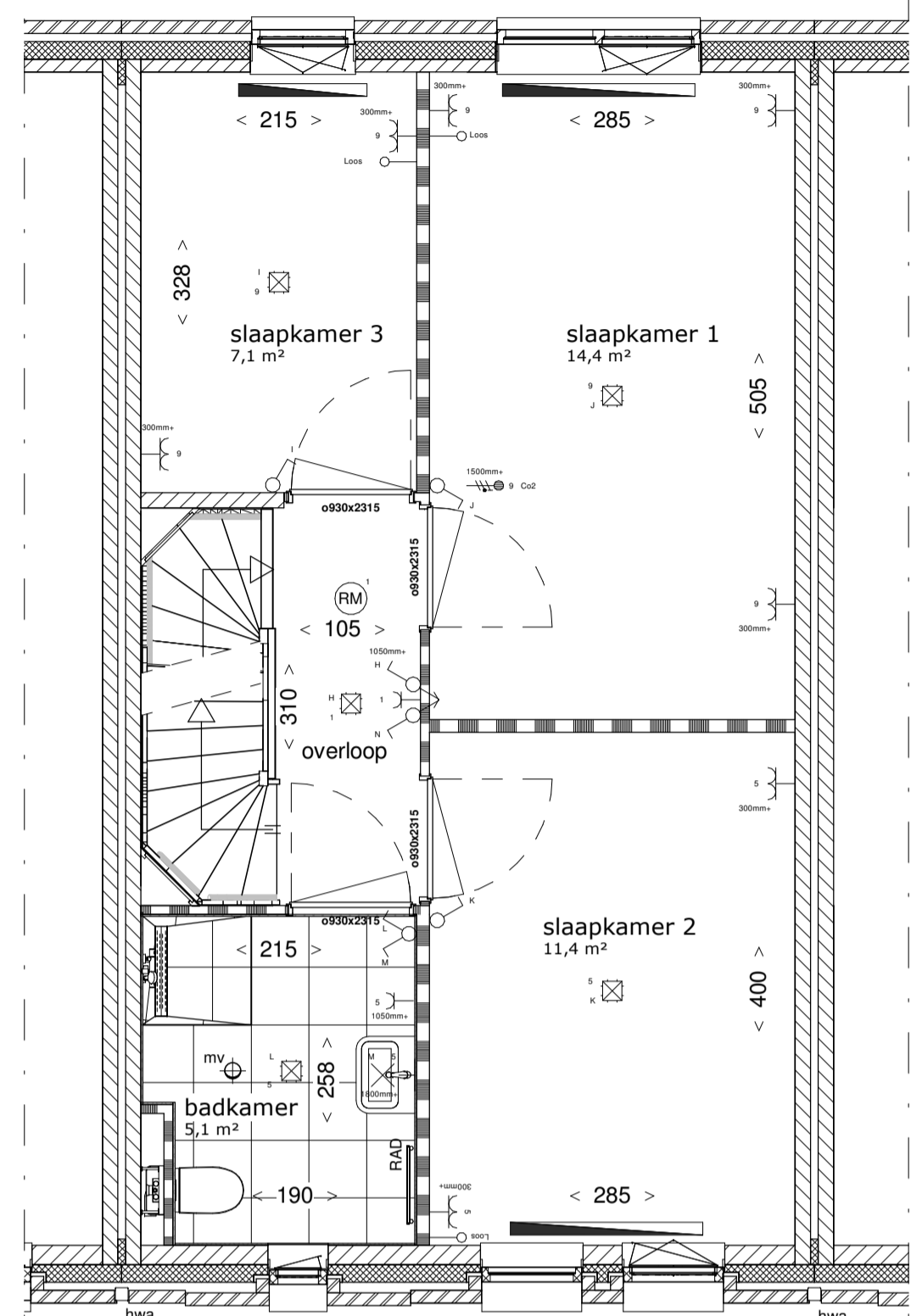
eerste verdieping 1 : 50
