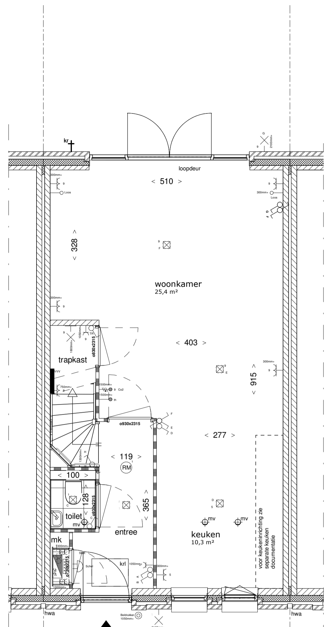
begane grond 1 : 50
