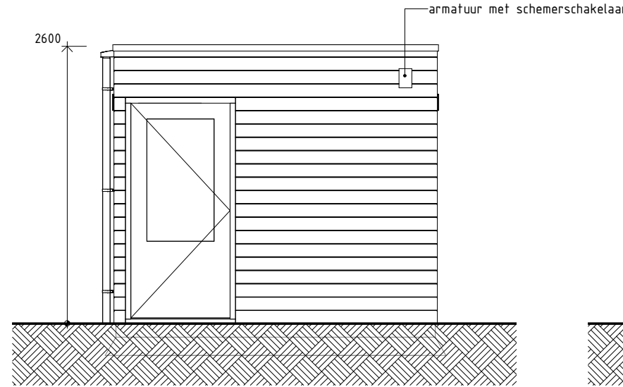
ZIJGEVEL RECHTS 1 : 50
