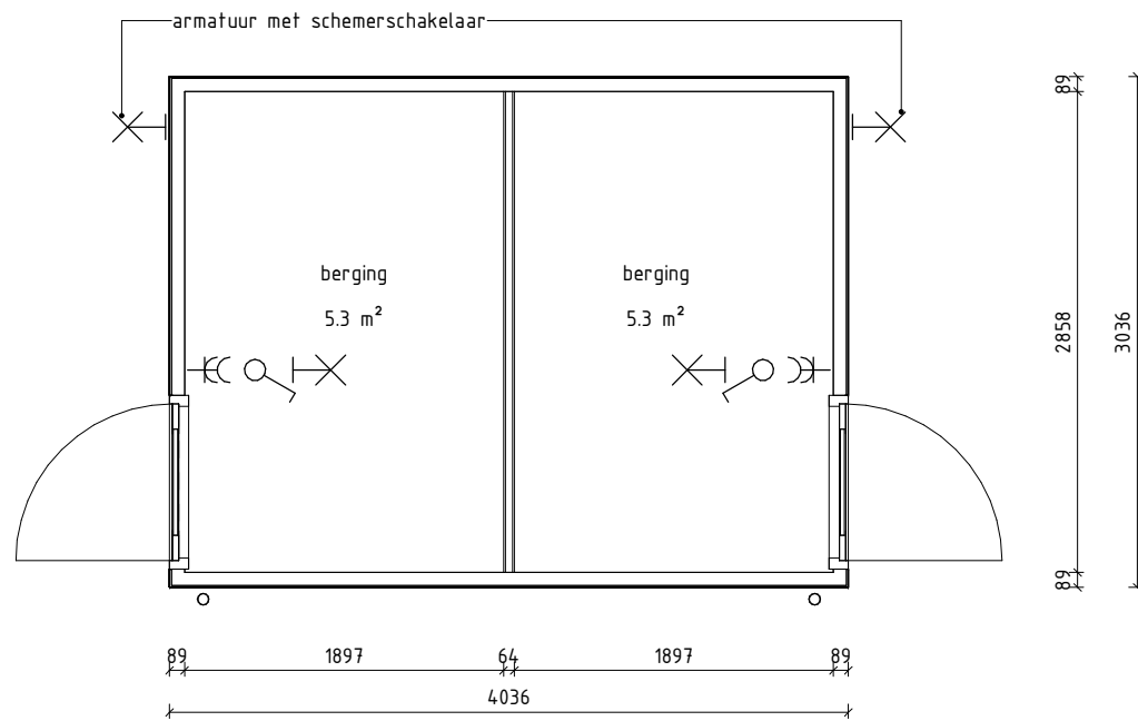
PLATTEGROND 1 : 50
