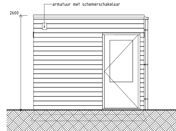
ZIJGEVEL LINKS 1 : 50
