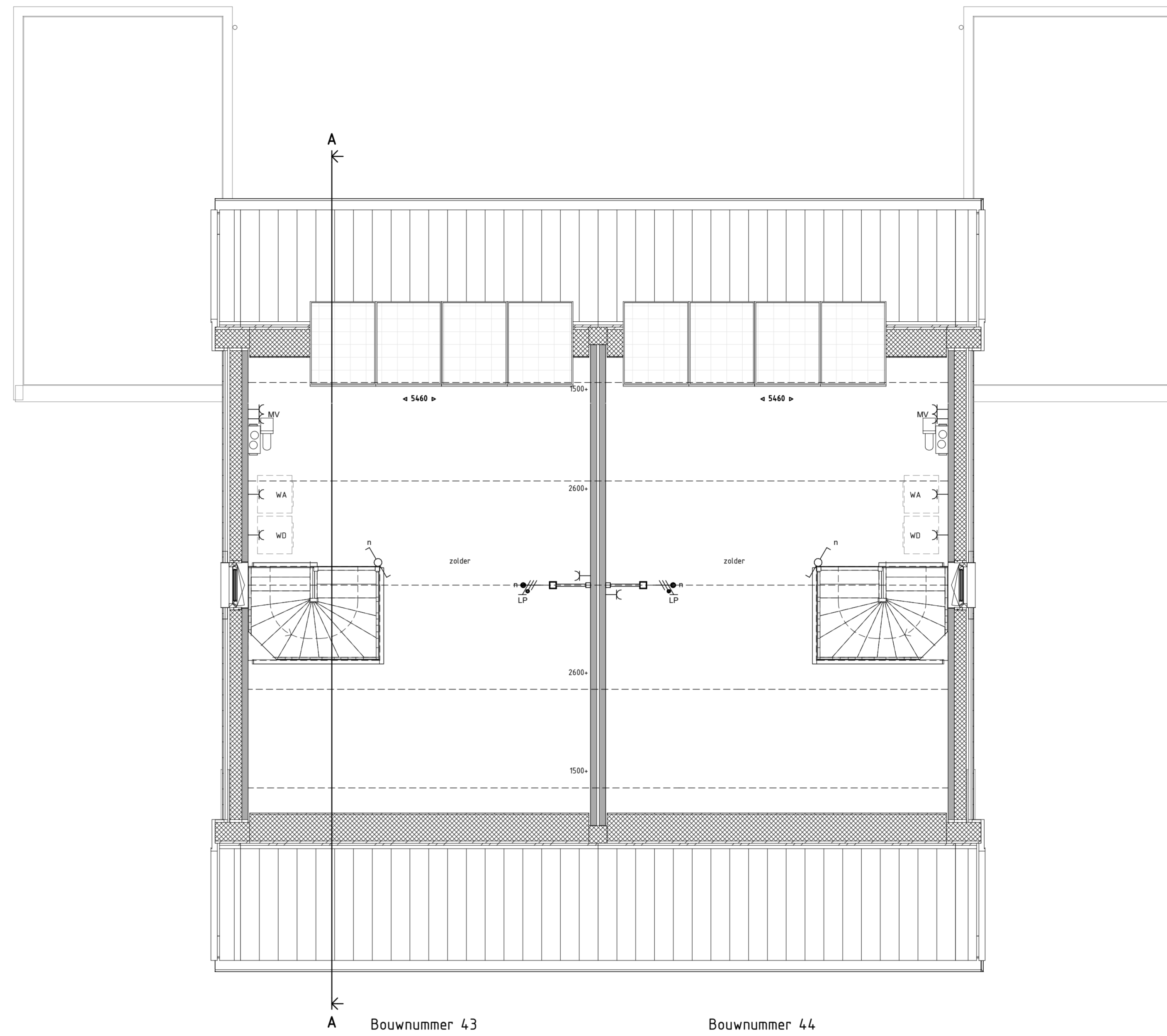
2E VERDIEPING 1 : 50
