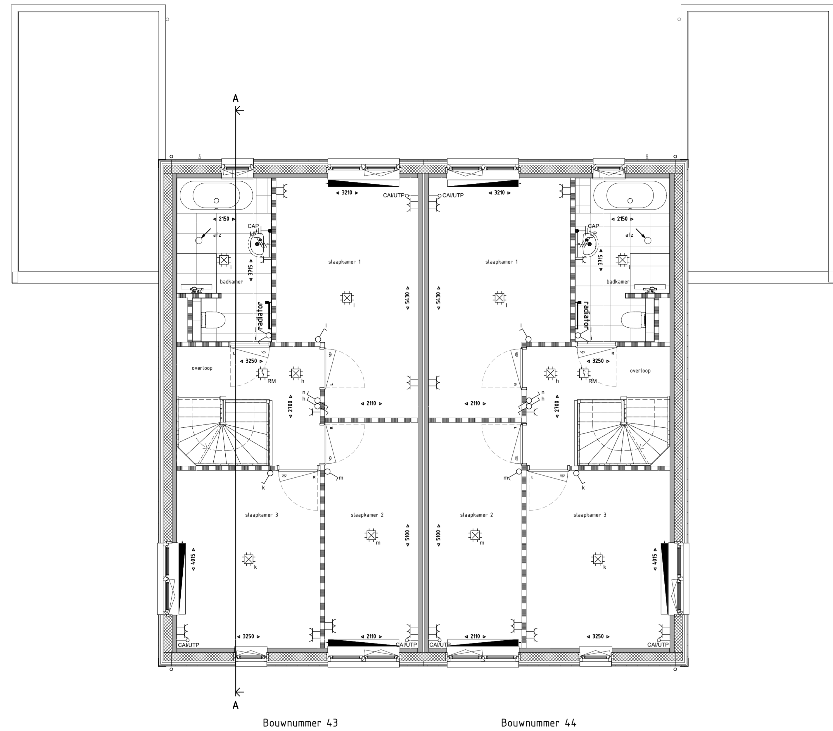
1E VERDIEPING 1 : 50
