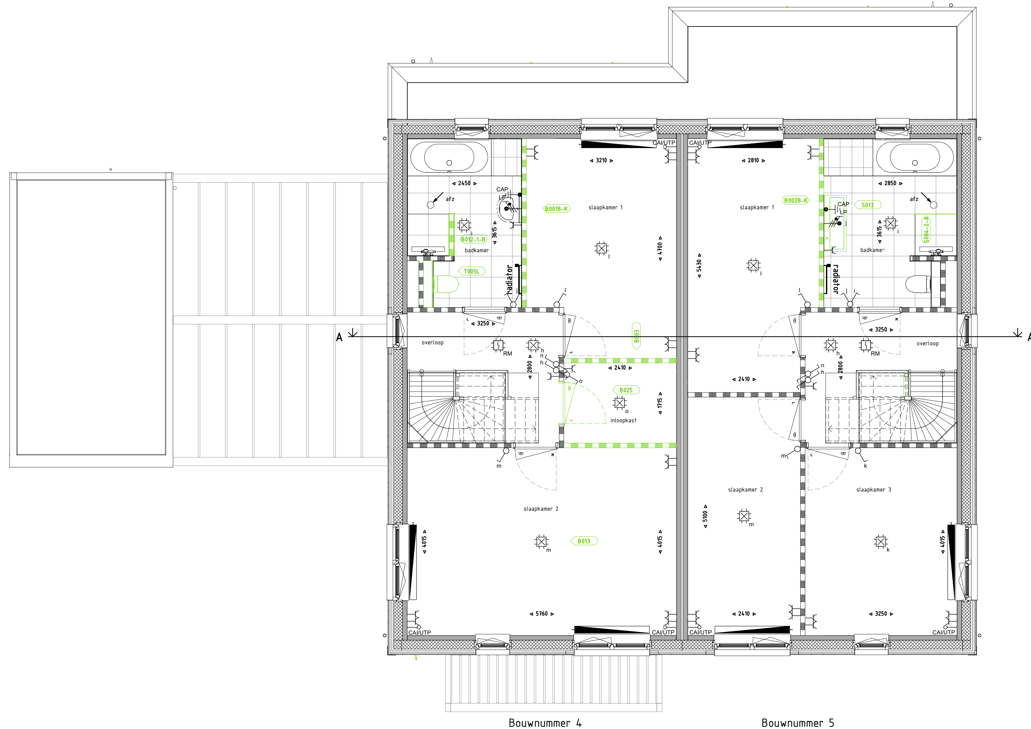
1E VERDIEPING 1 : 50
