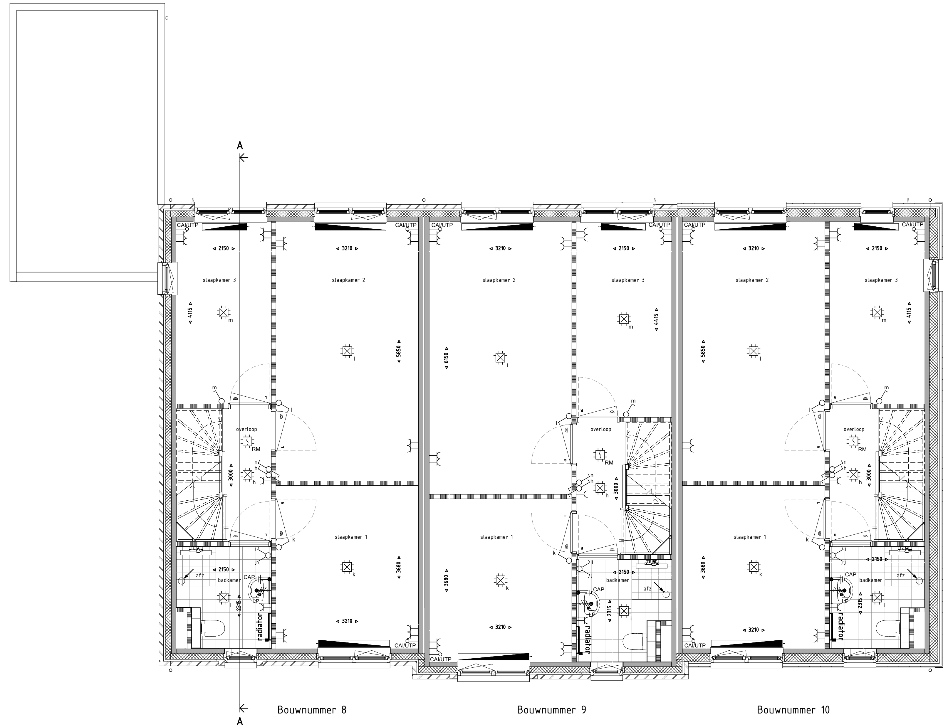
1E VERDIEPING 1 : 50
