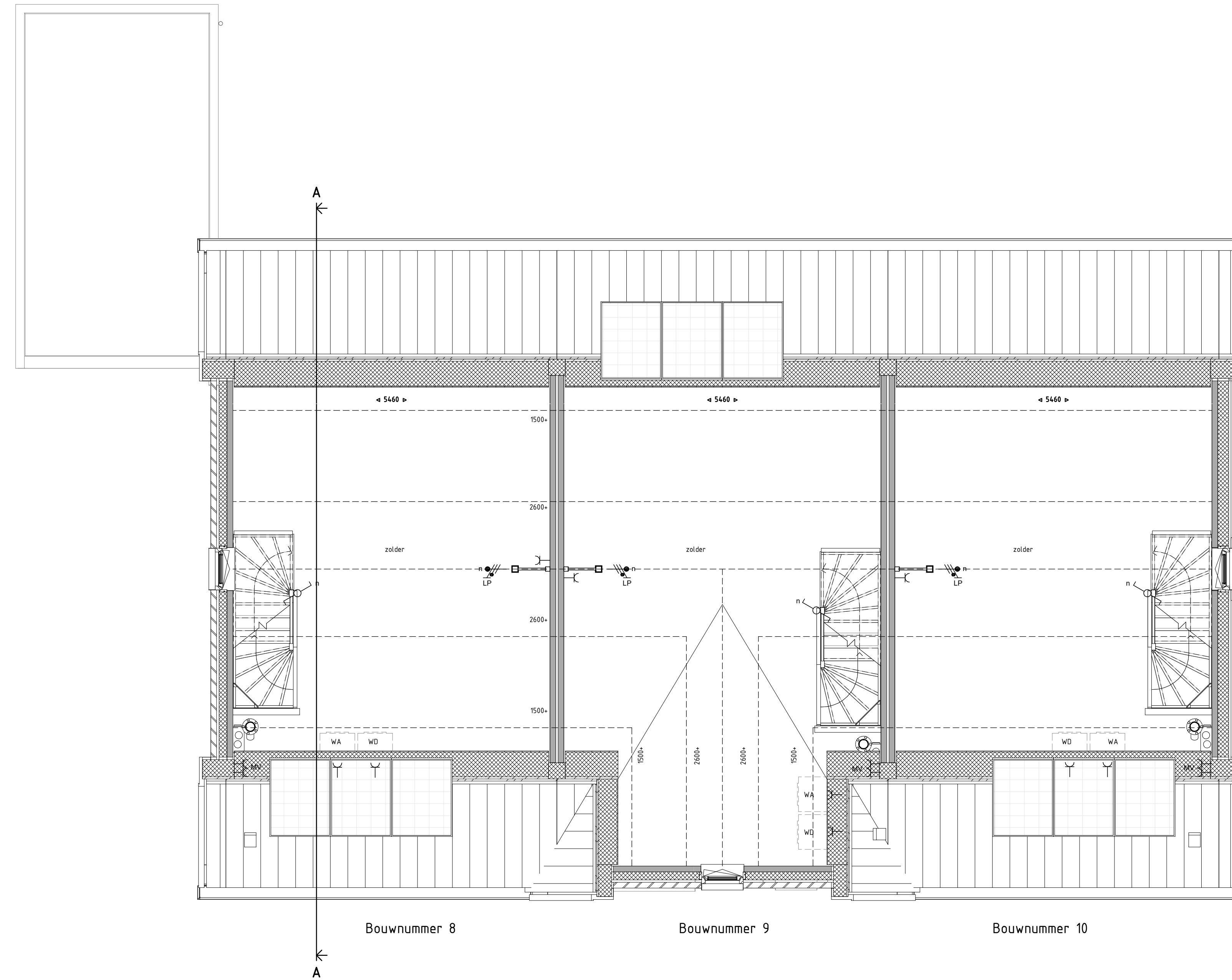
2E VERDIEPING 1 : 50
