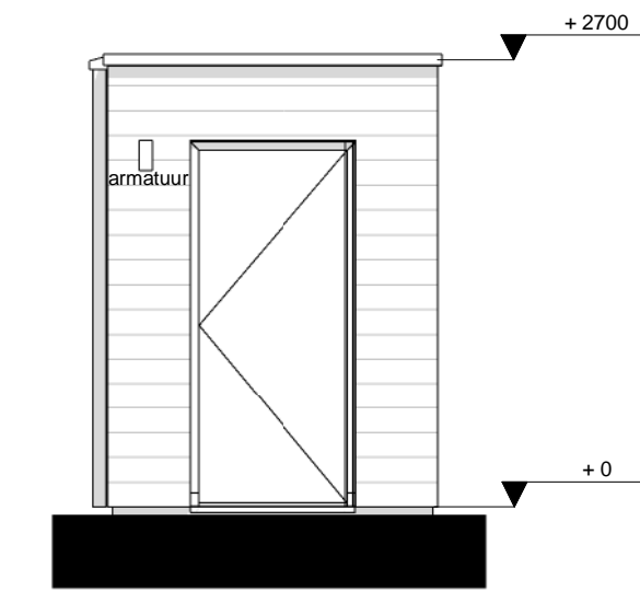
rechtgevel
