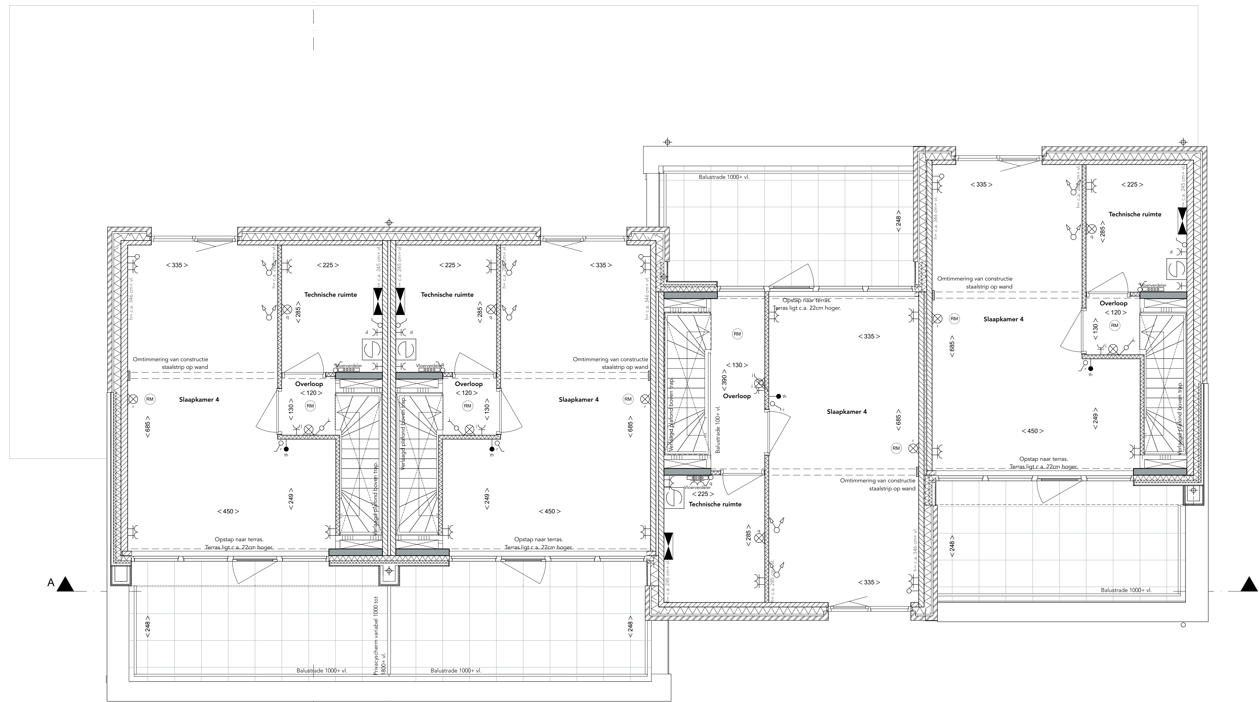
3e verdieping Schaal 1:50
