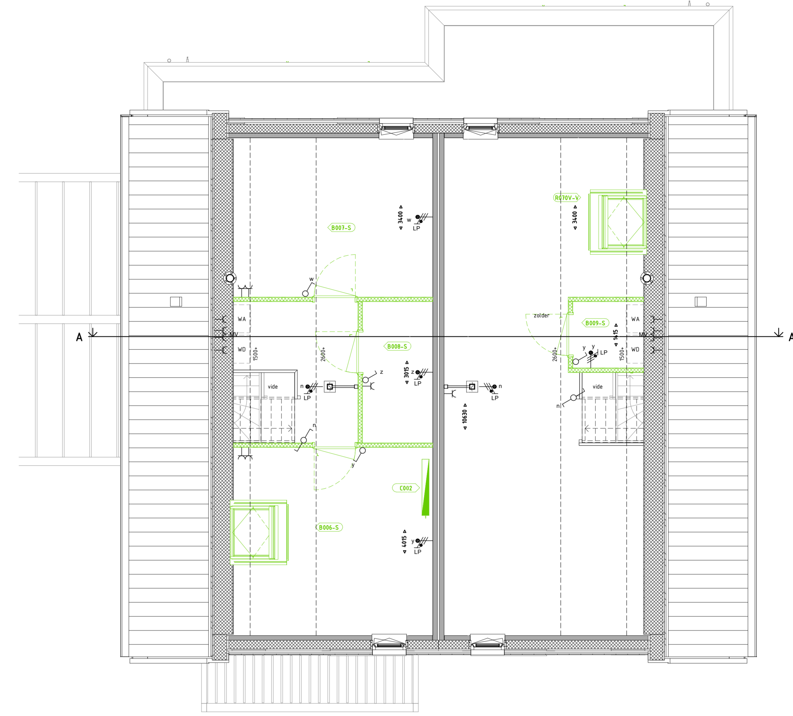
2E VERDIEPING 1 : 50
