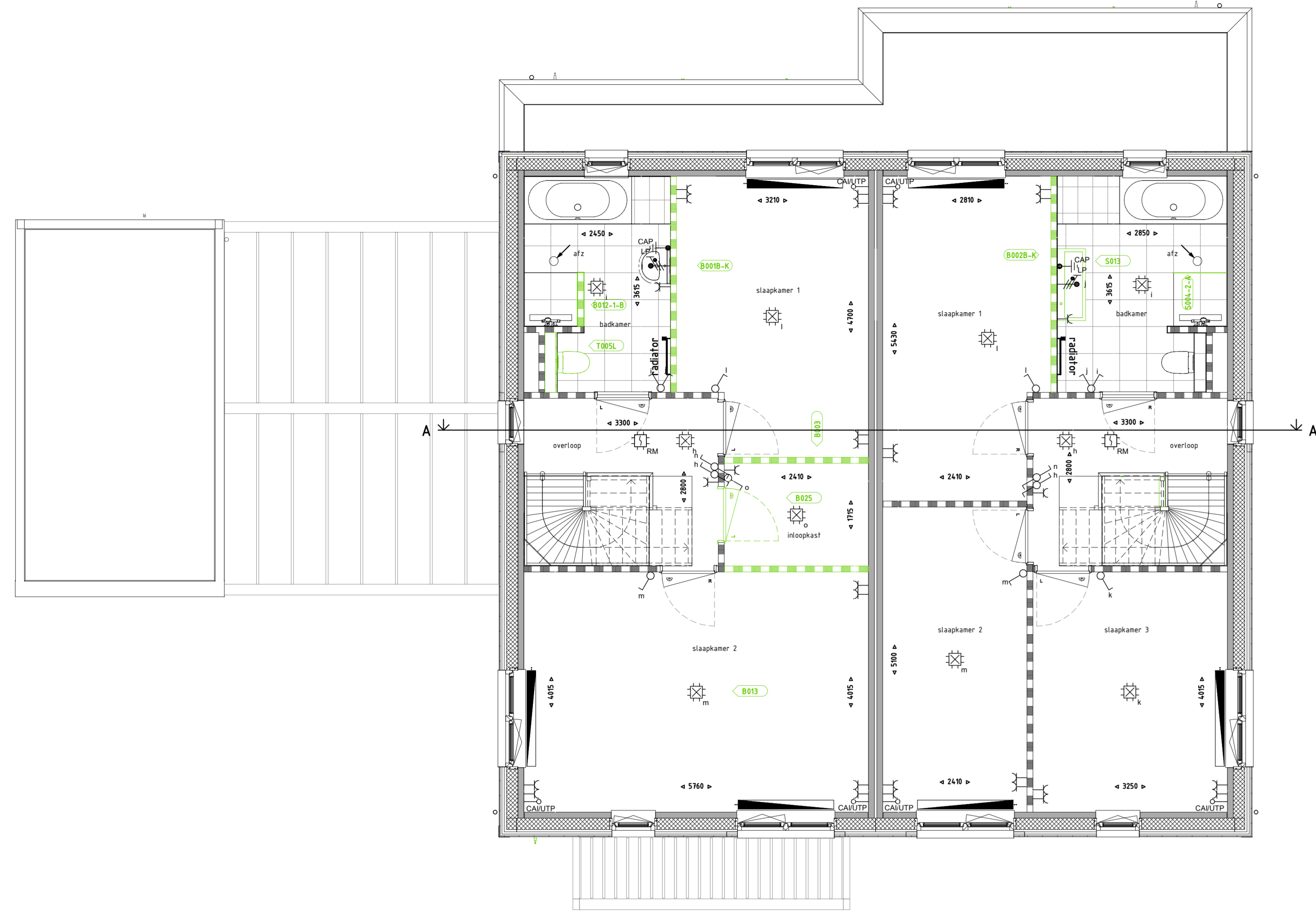
1E VERDIEPING 1 : 50
