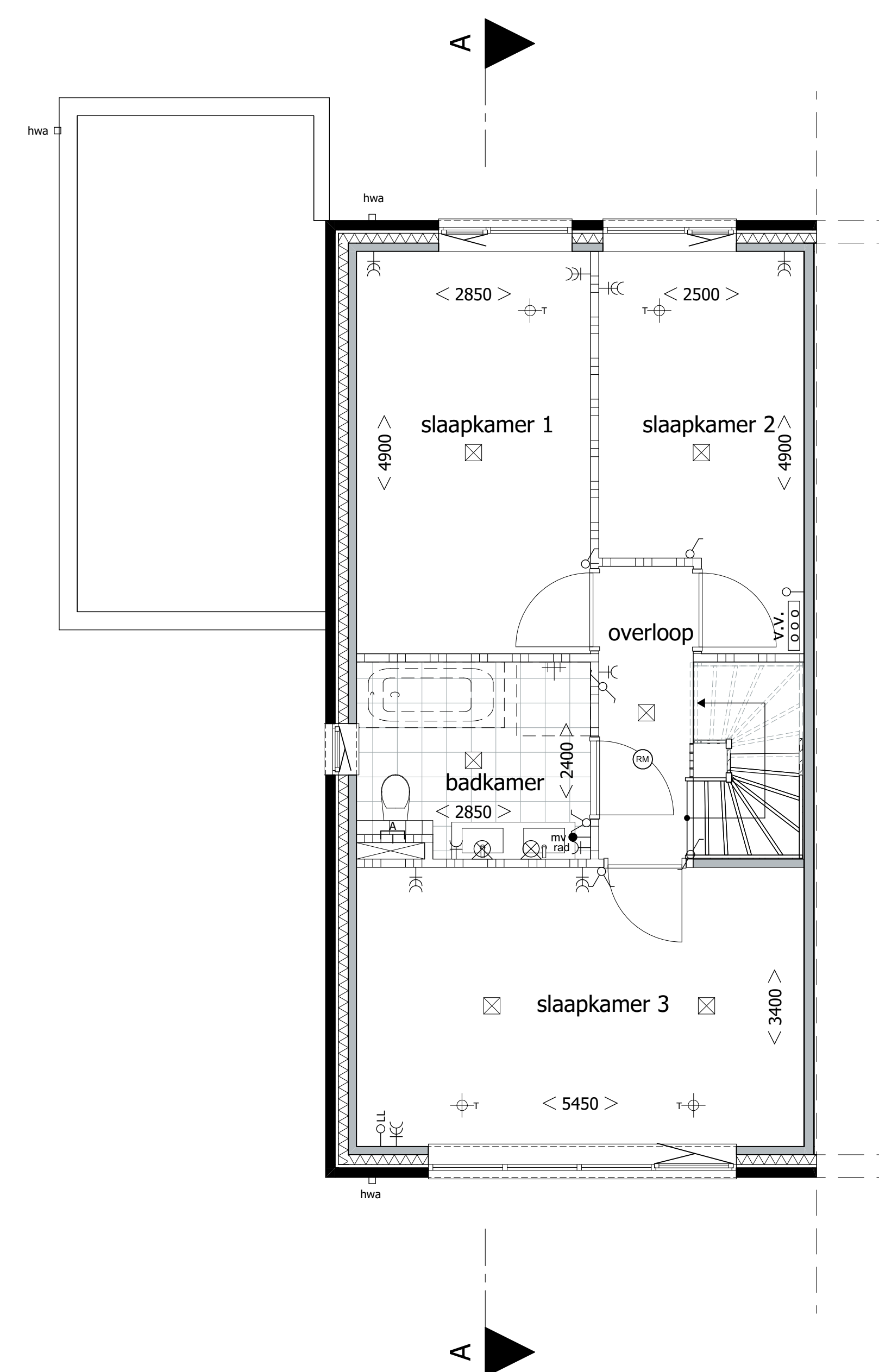
Verdieping 1 type D1
