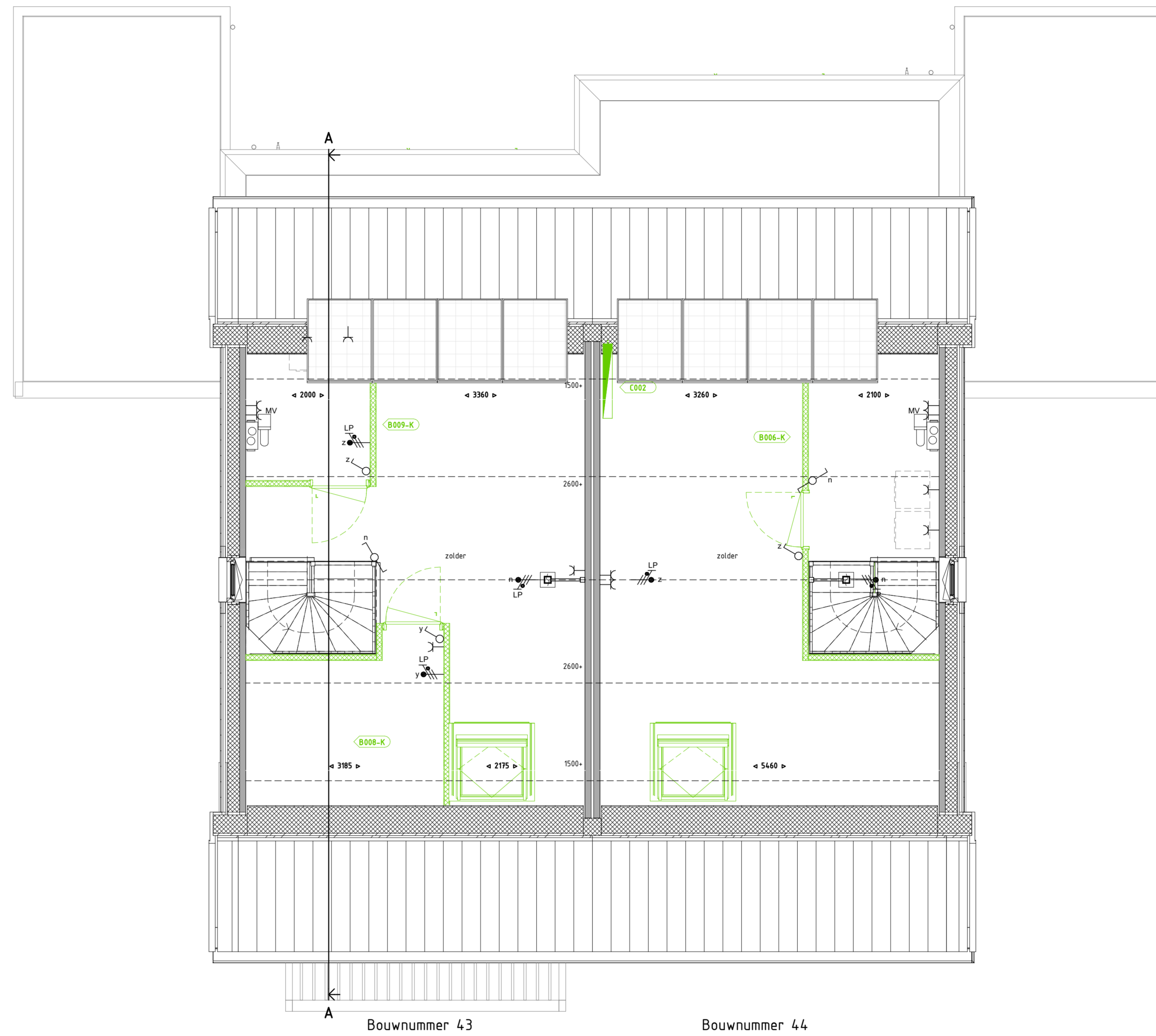
2E VERDIEPING 1 : 50
