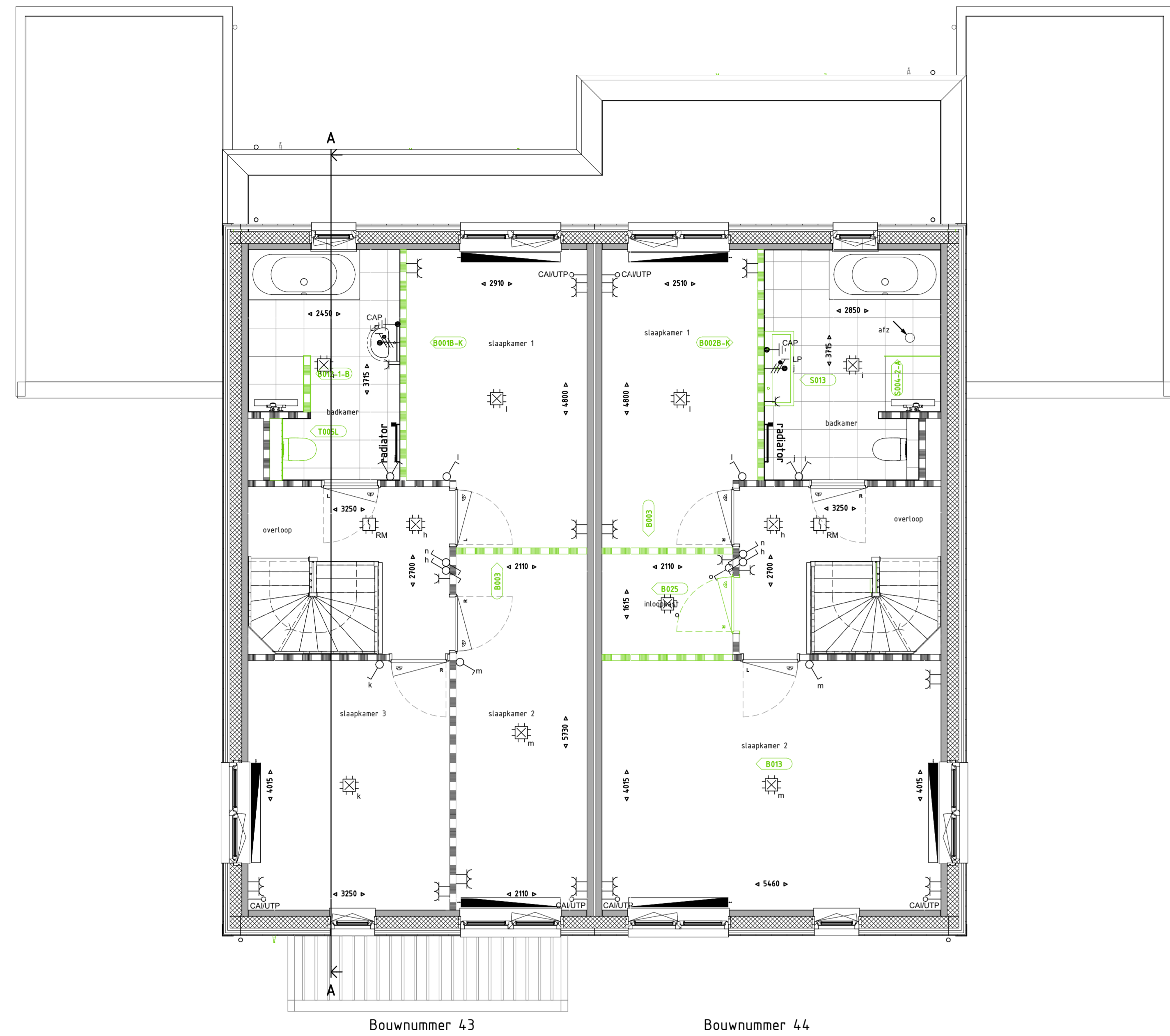
1E VERDIEPING 1 : 50
