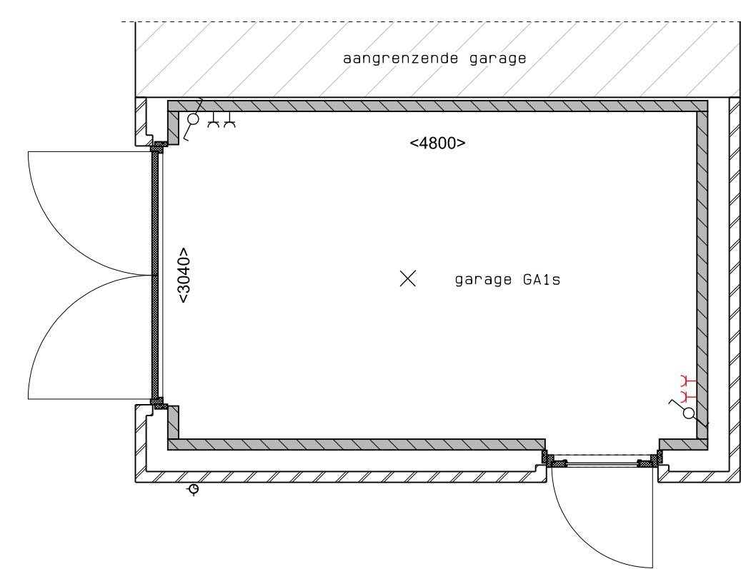
plattegrond
