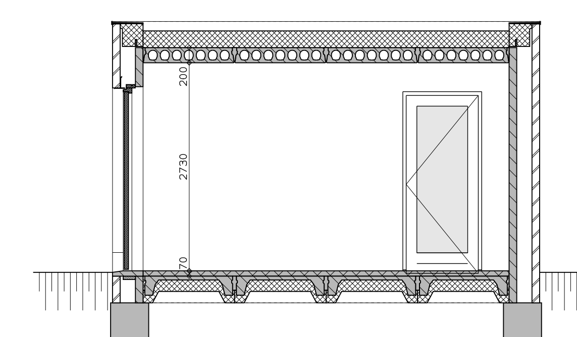
doorsnede
