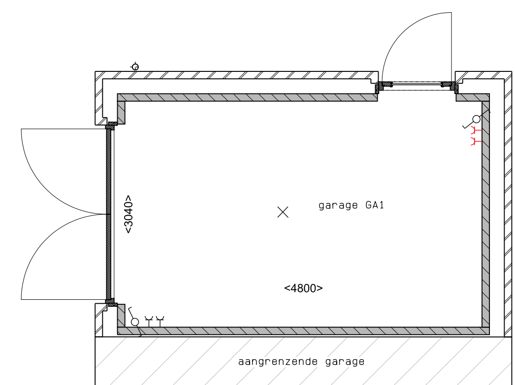
plattegrond
