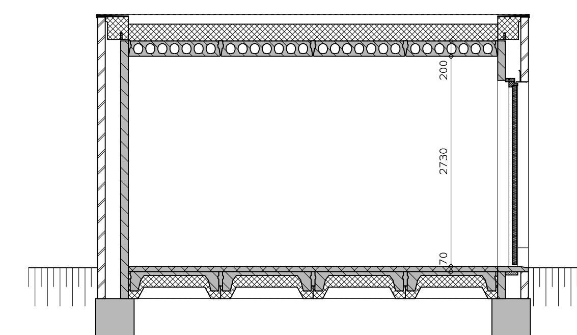
doorsnede
