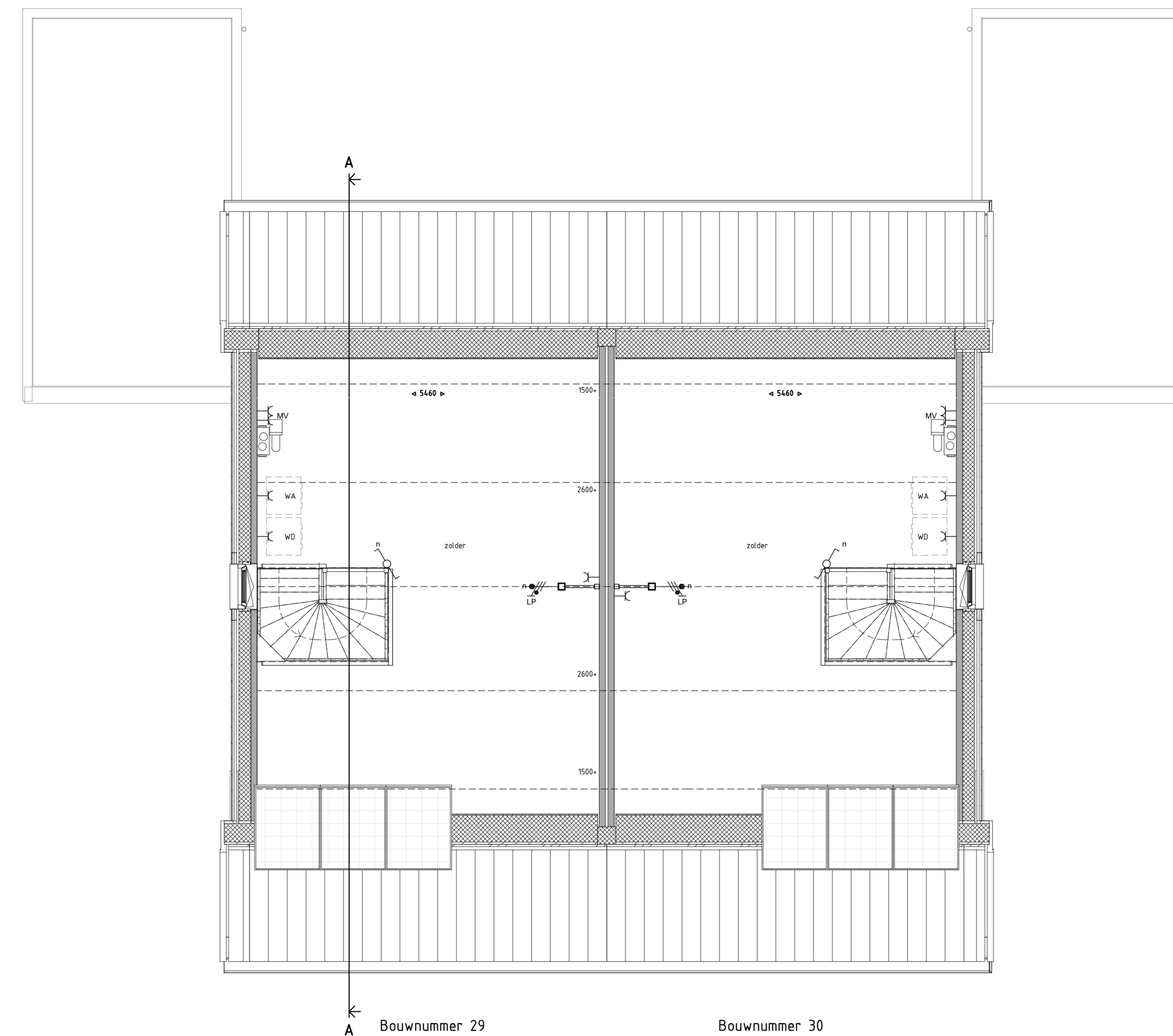
2E VERDIEPING 1 : 50
