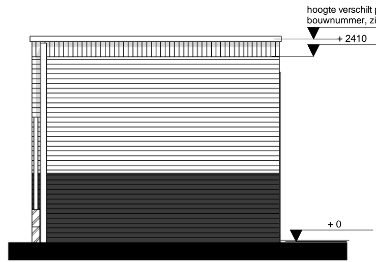
voorgevel
