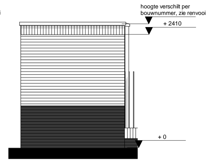
linksgevel
