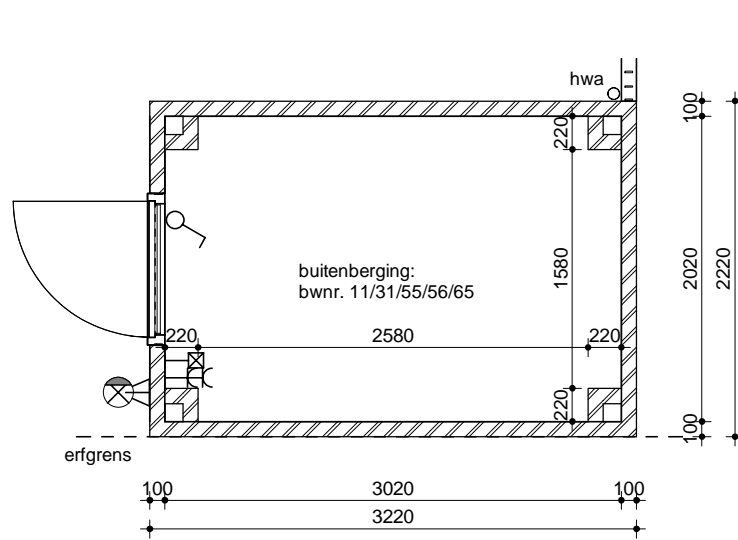
begane grond
