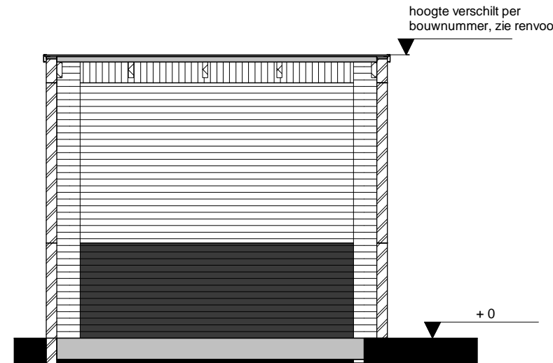
langsdoorsnede
