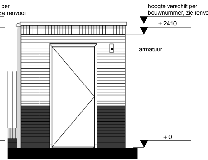
rechtgevel
