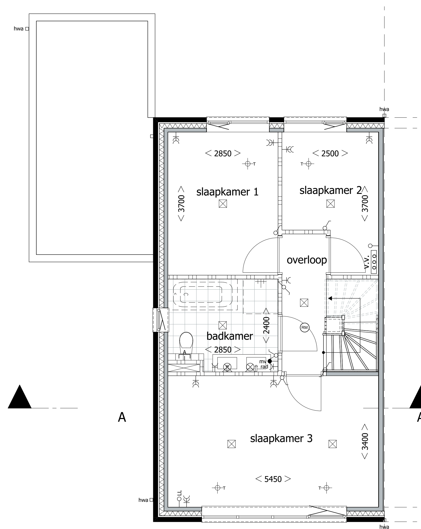
Verdieping 1 type D2
