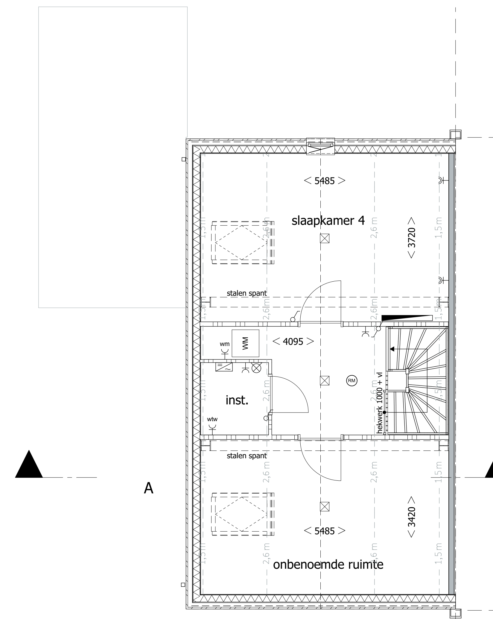
Verdieping 2 type D2
