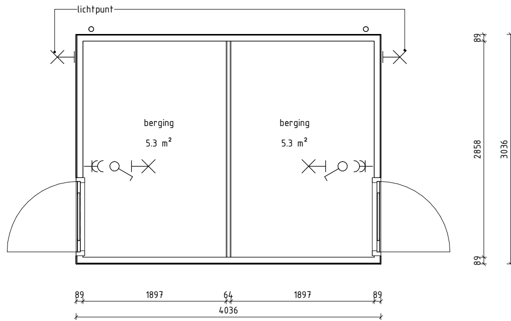
PLATTEGROND 1 : 50
