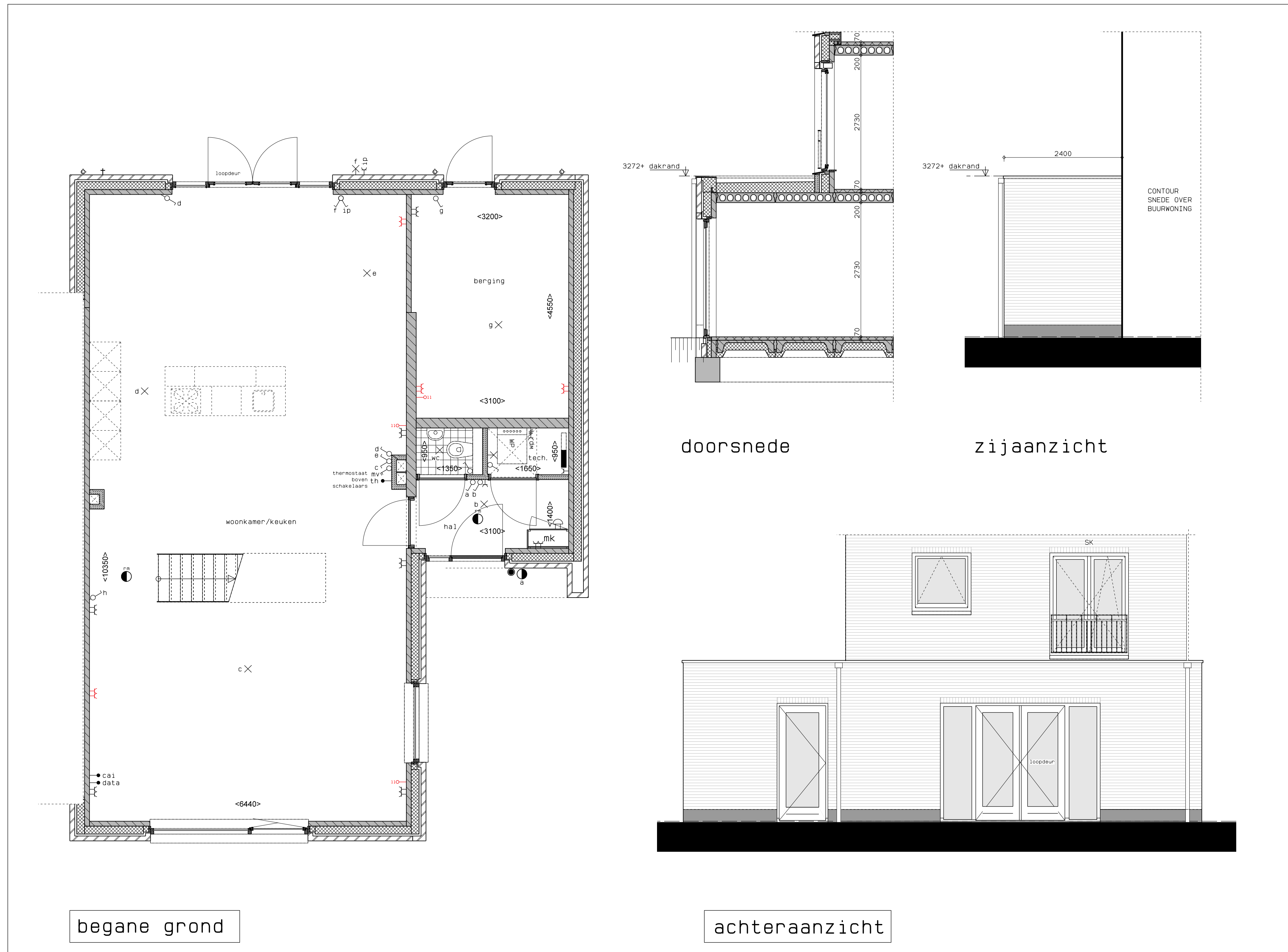
Type 6.7Eb-5, Uitbouw achter 2,4 m, kavel 62
