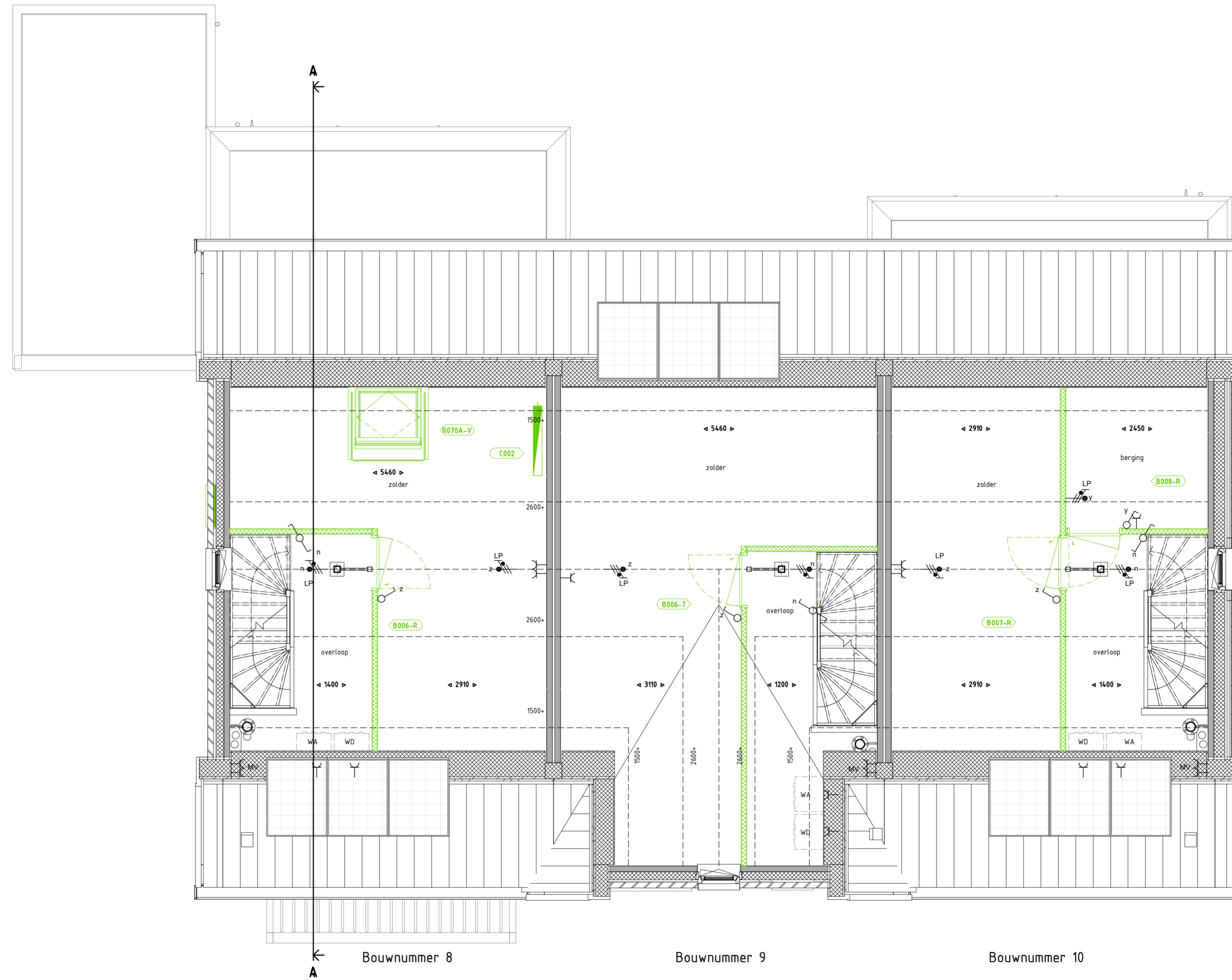
2E VERDIEPING 1 : 50
