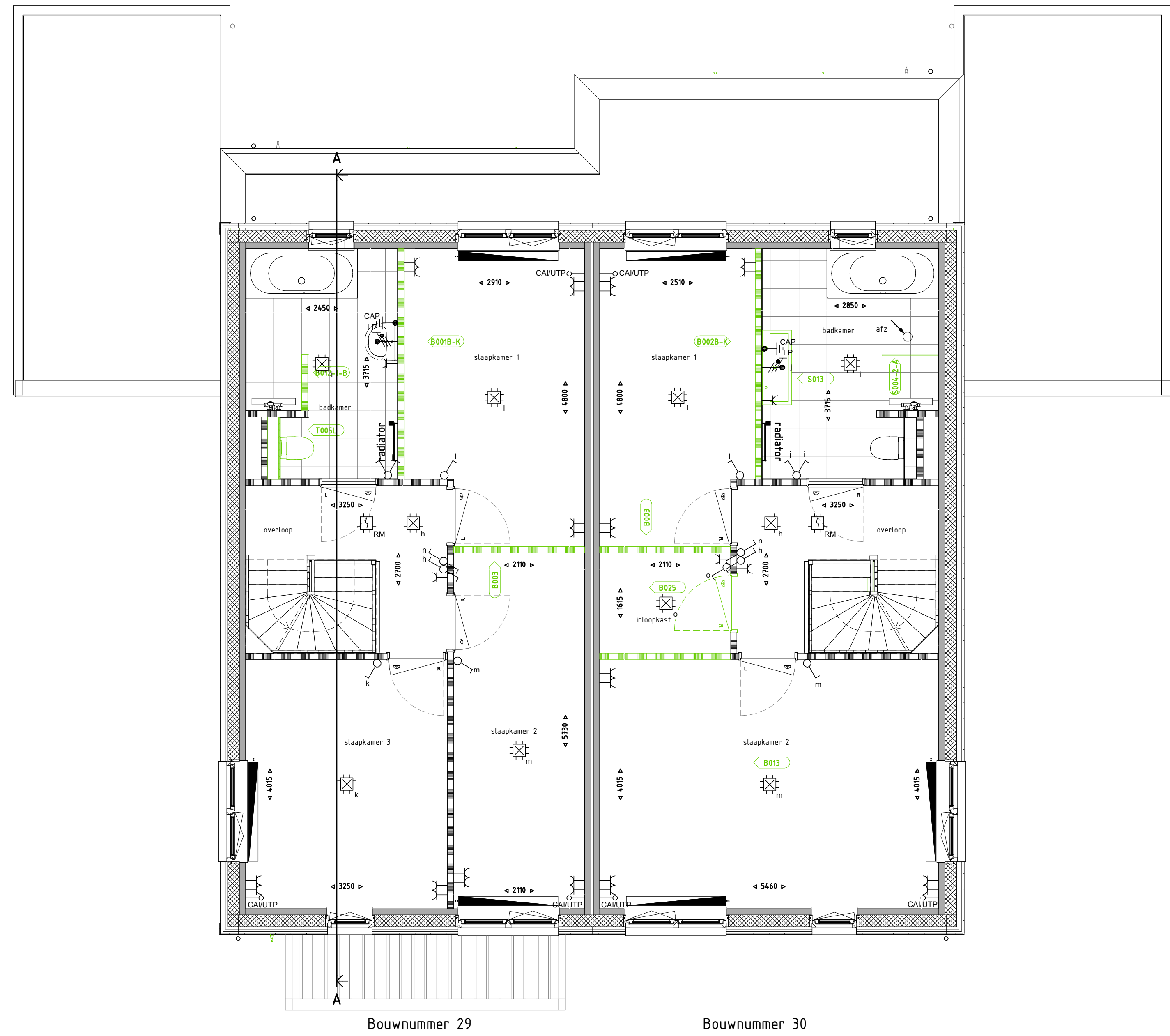
1E VERDIEPING 1 : 50
