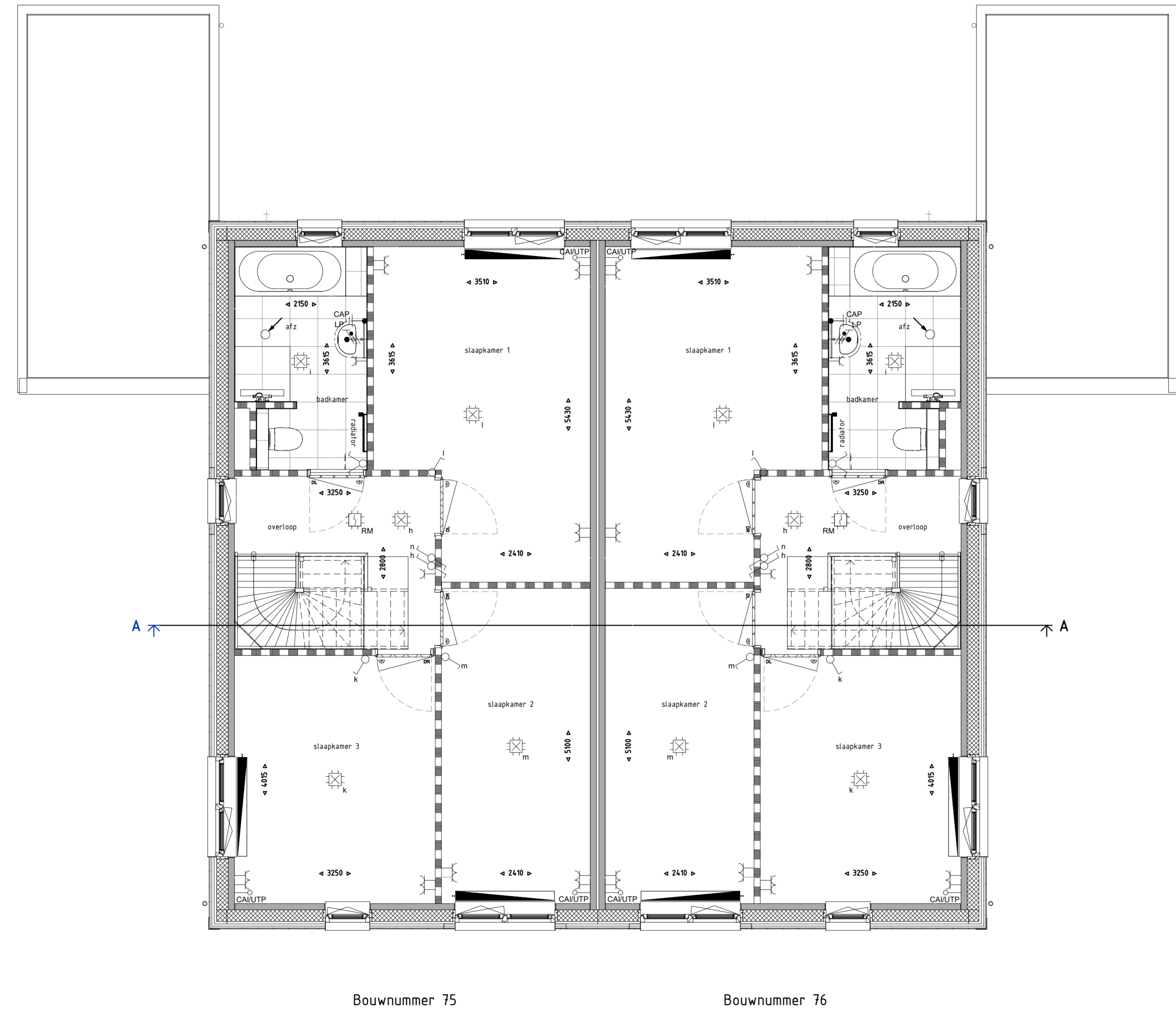
1E VERDIEPING 1 : 50
