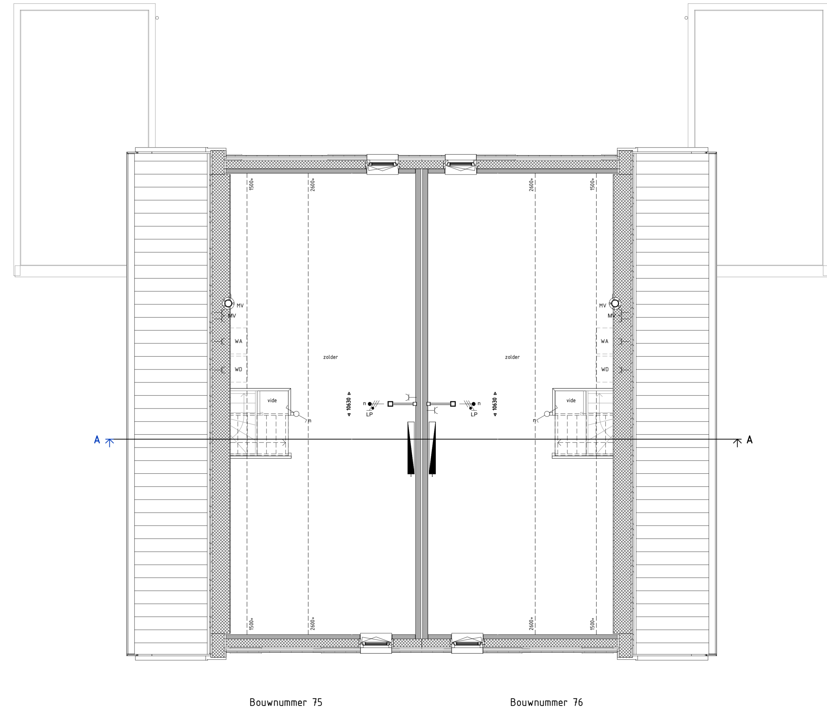
2E VERDIEPING 1 : 50
