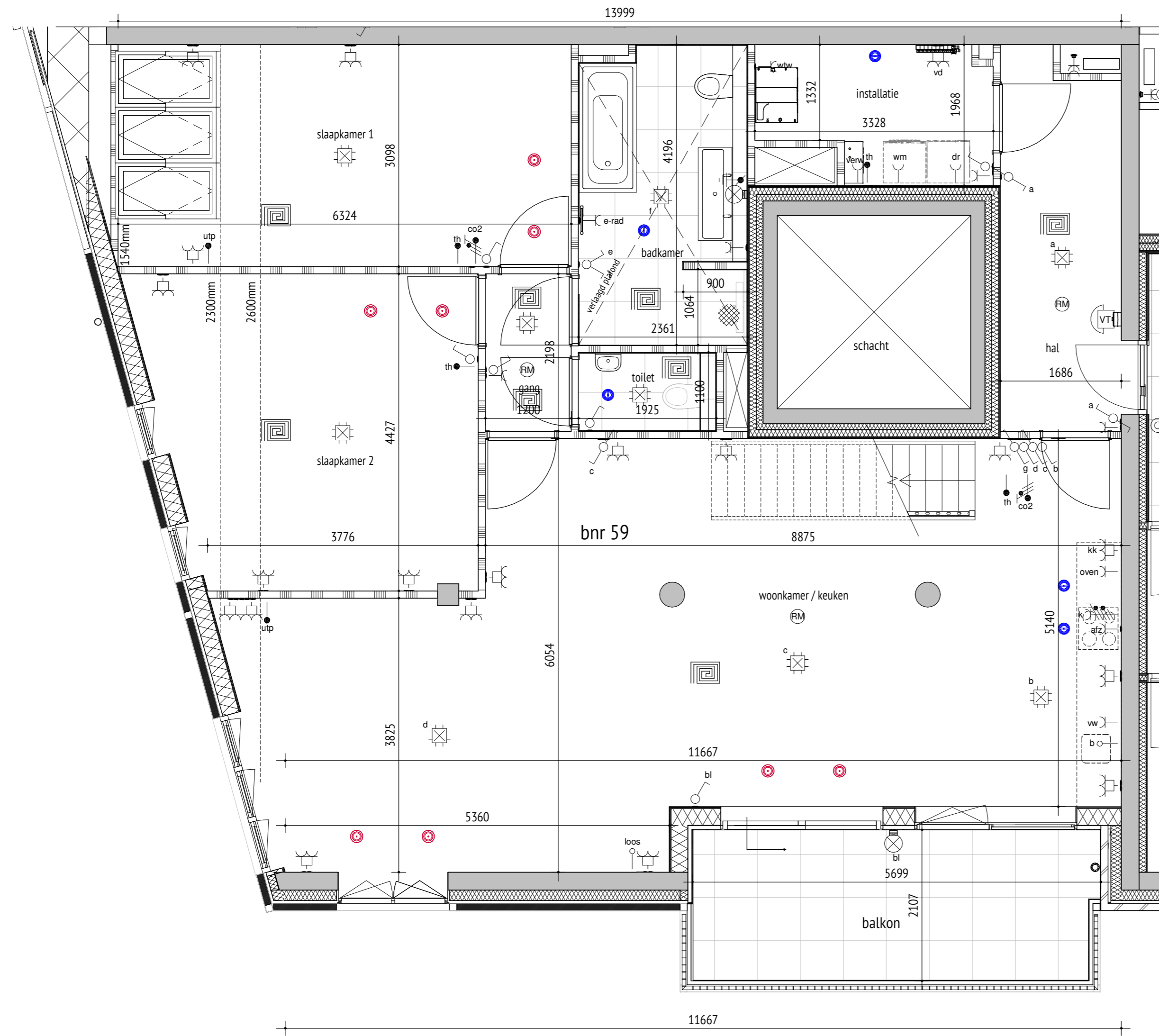
Bnr. 59 - 5de verdieping type B2
