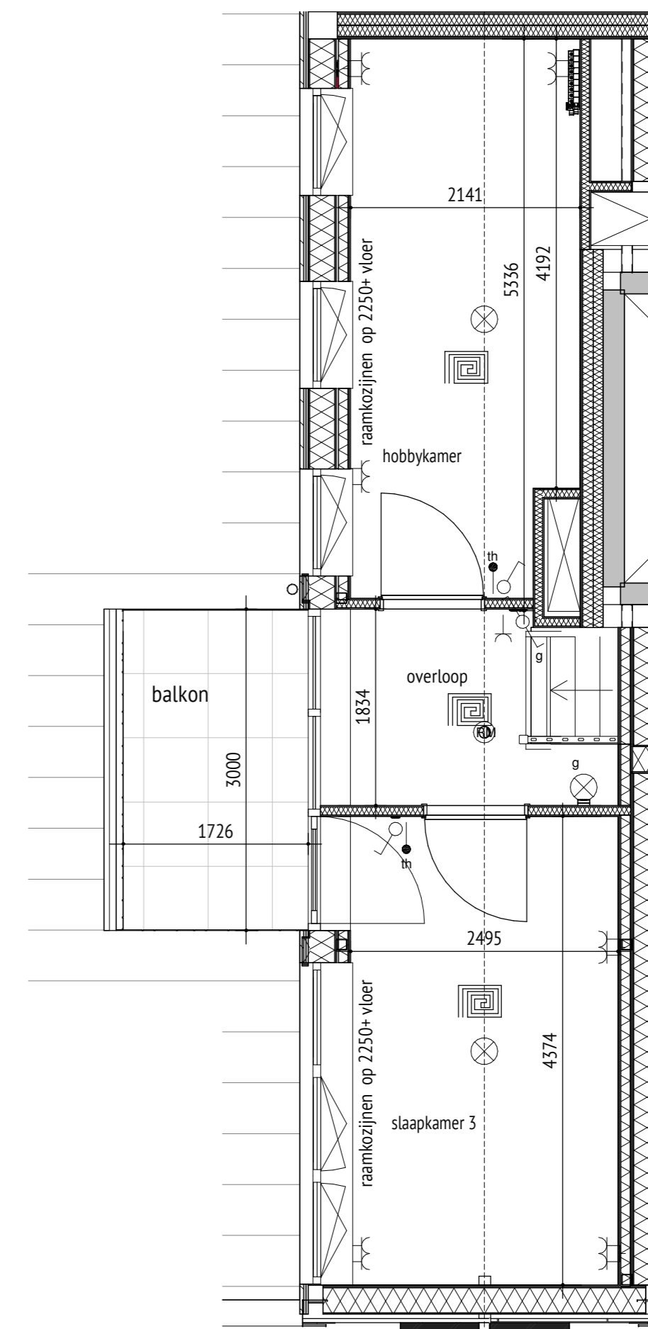
Bnr. 59 - 6de verdieping
