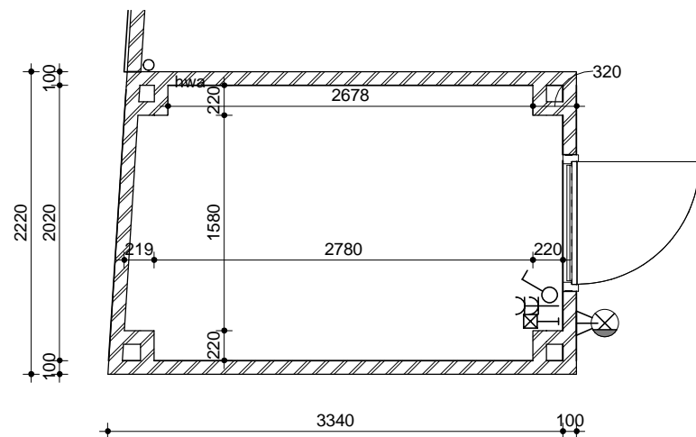
begane grond
