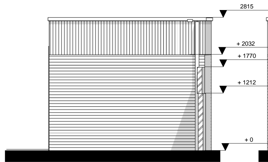
voorgevel
