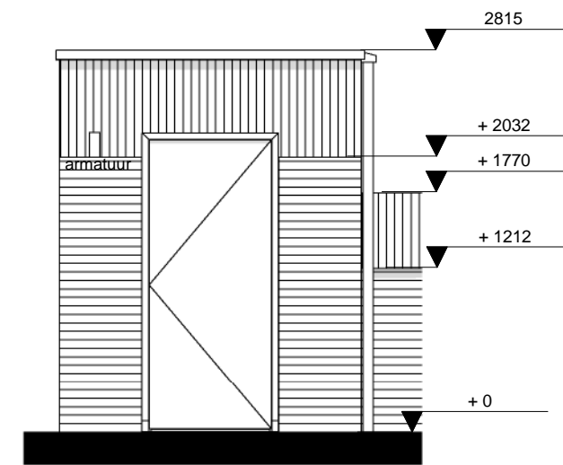
linksgevel
