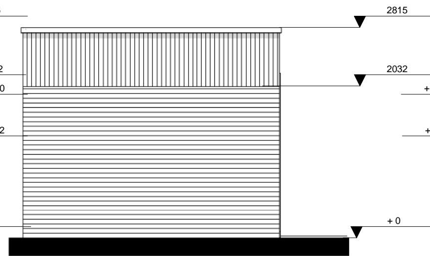
achtergevel
