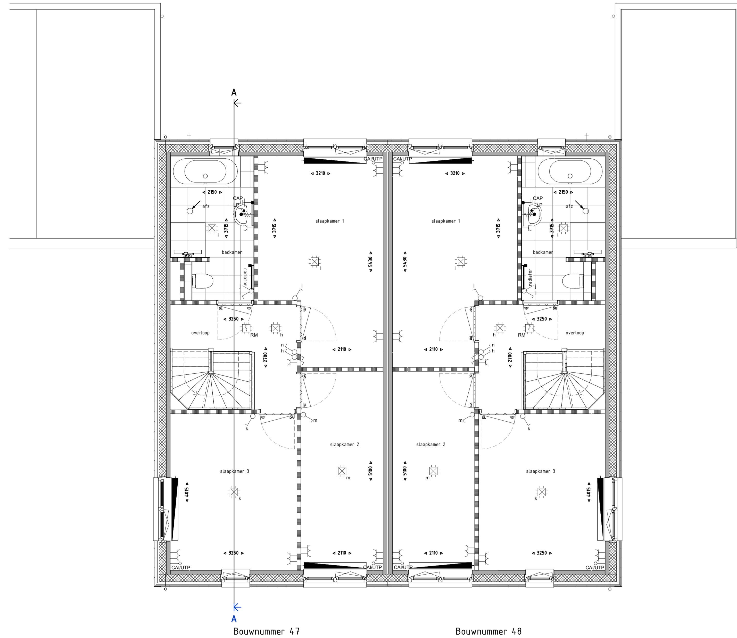
1E VERDIEPING 1 : 50
