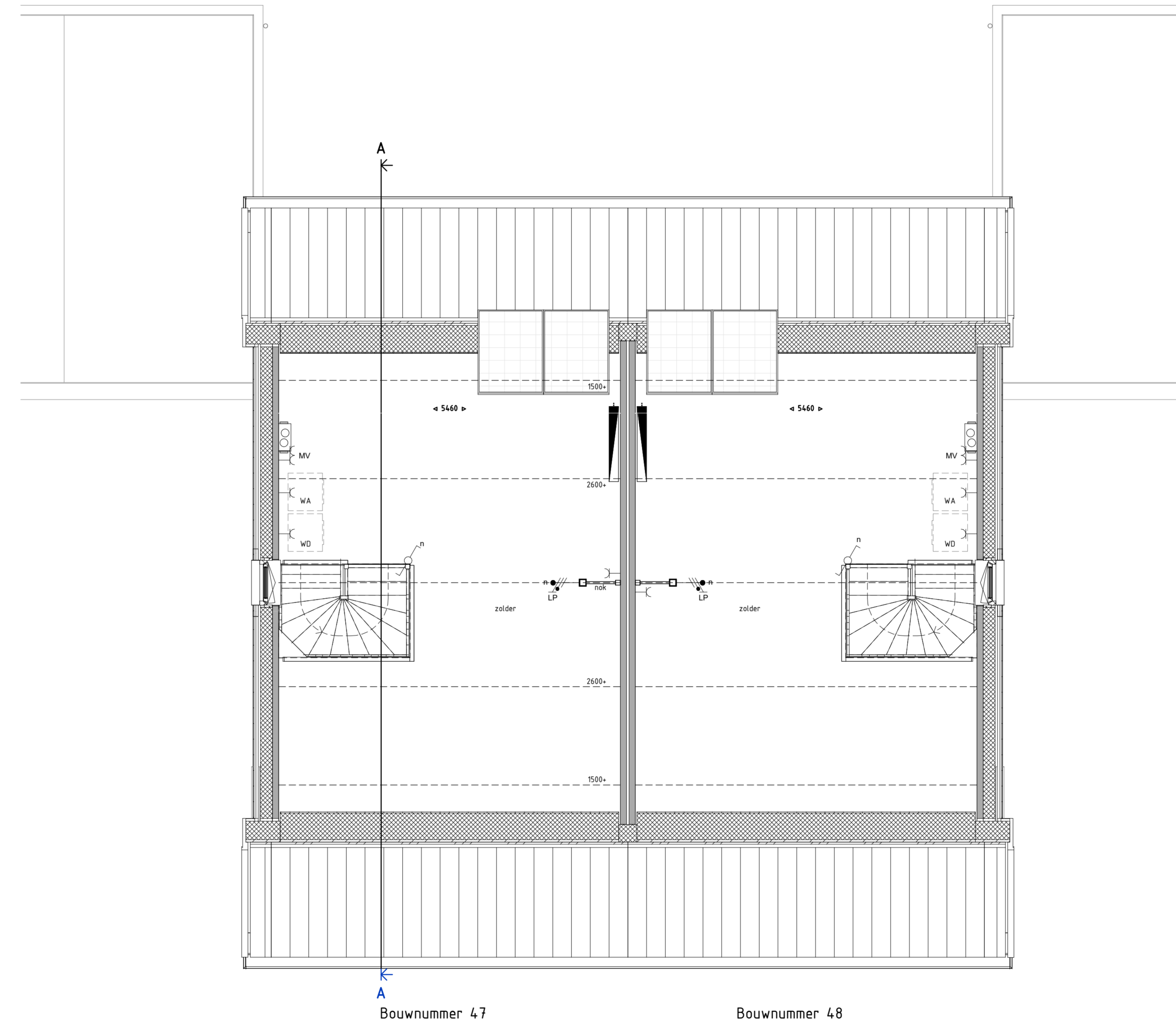
2E VERDIEPING 1 : 50
